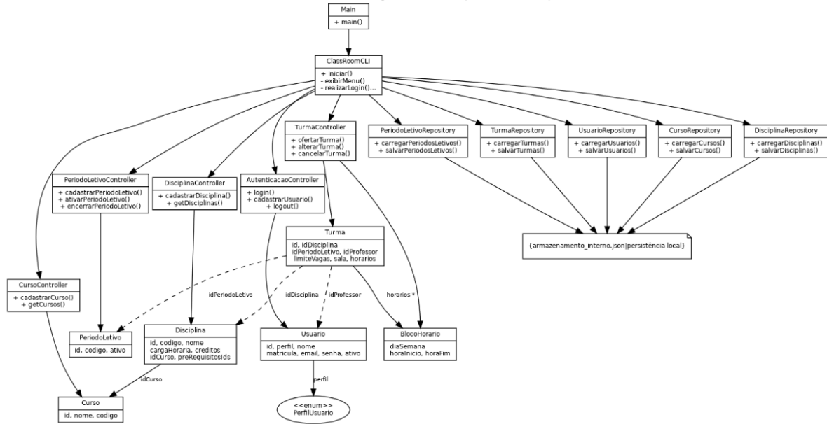
ClassRoomPB — Diagrama de Classes (visão de camadas)
