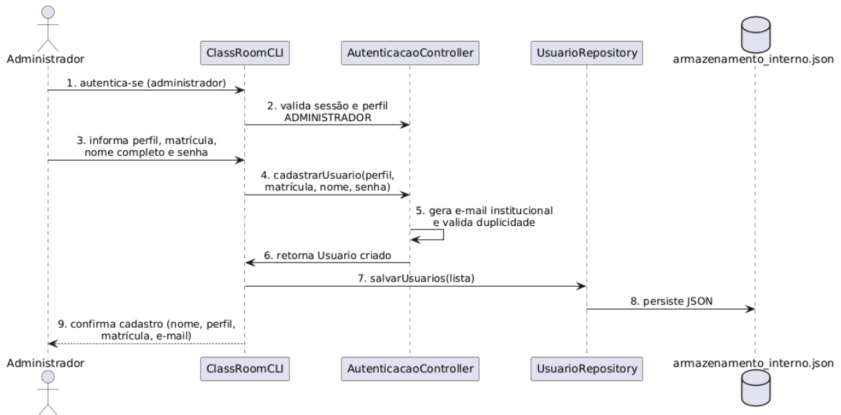
ClassRoomPB — Sequência: Processo cadastral de usuários
