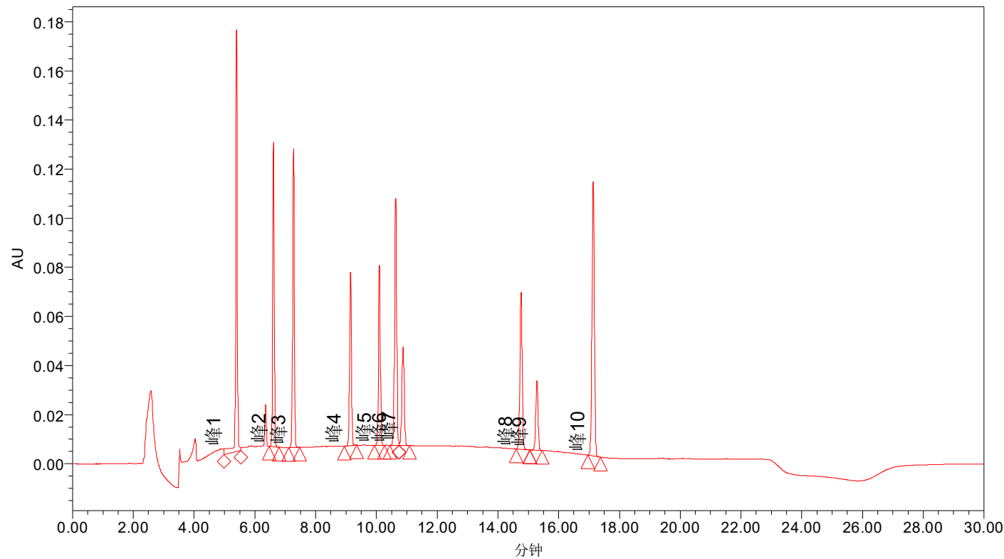
重叠色谱图
