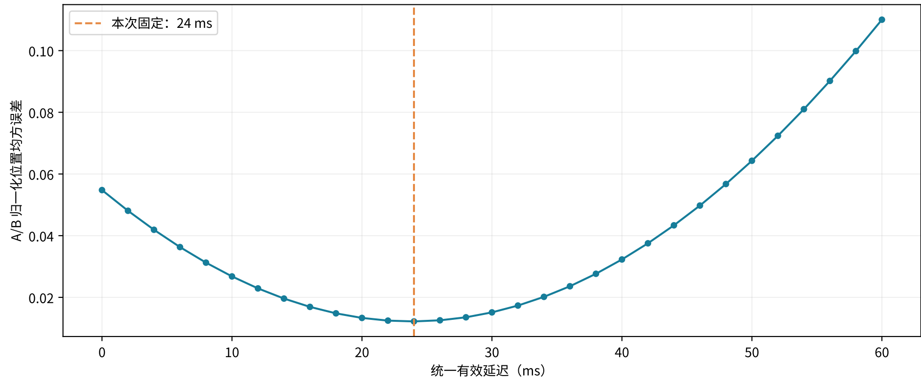
冻结六关节物理参数后的统一延迟检查
