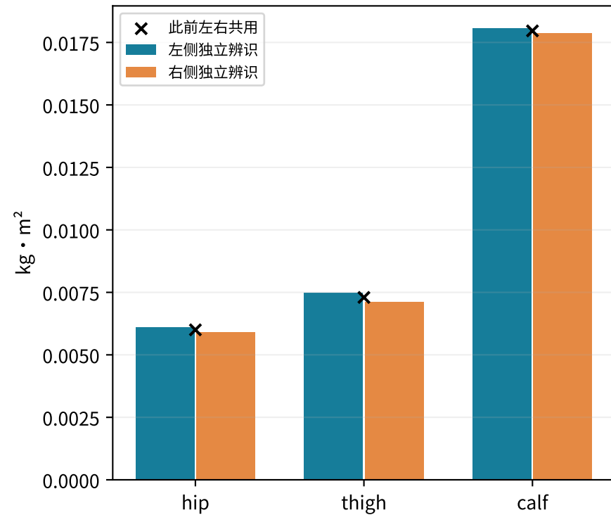
关节附加惯量 (armature)
