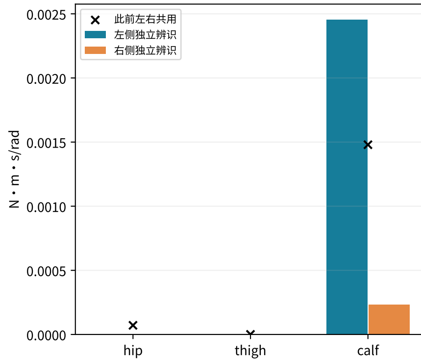
被动黏性阻尼
