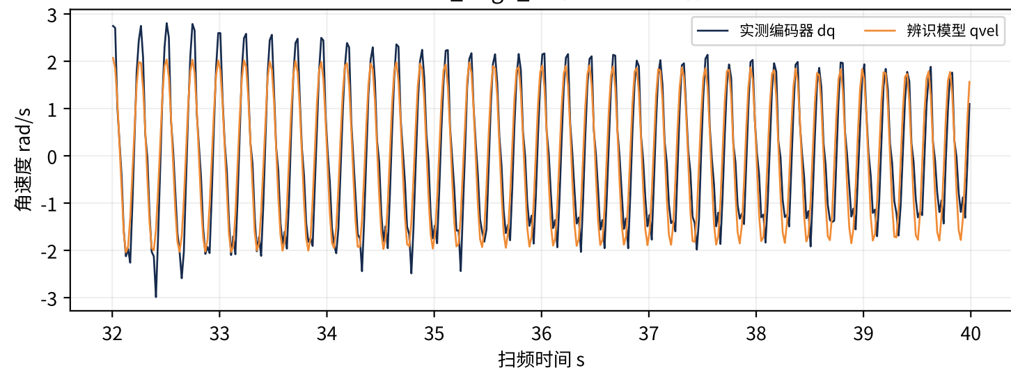
C 组 · L_calf_ · 高频段速度对照
