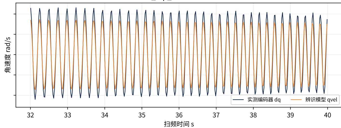
C 组 · R_thigh_ · 高频段速度对照
