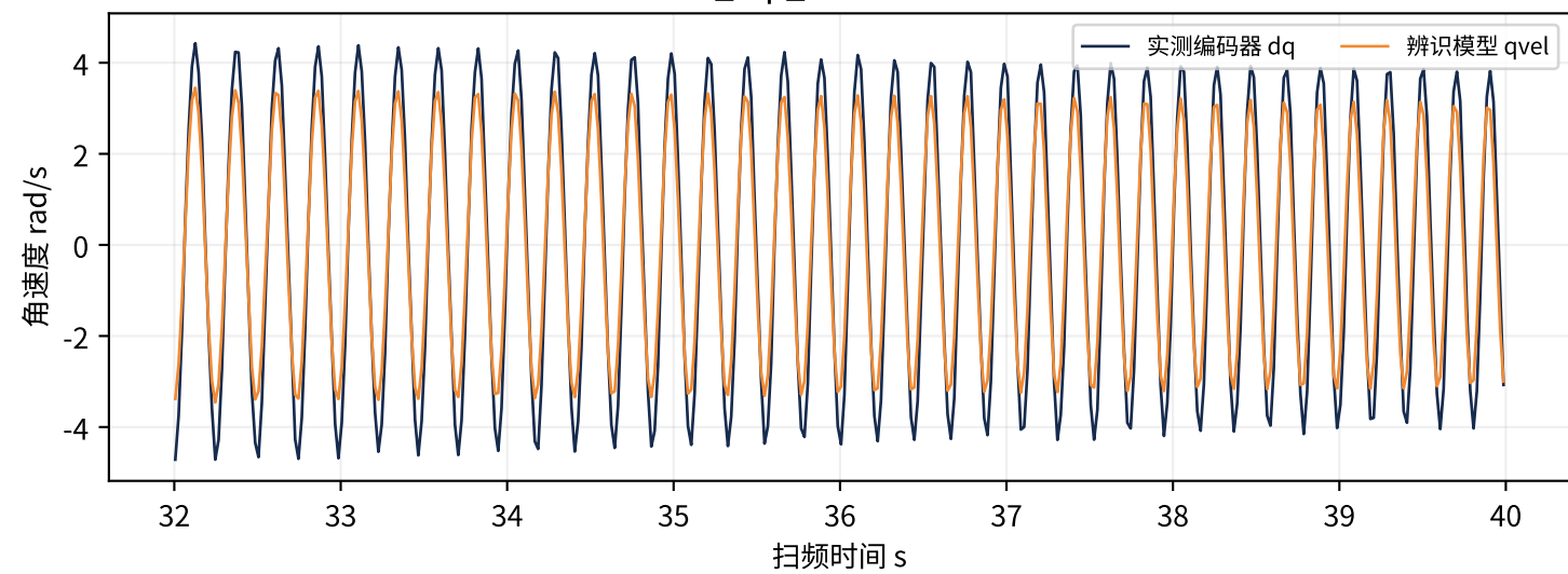
C 组 · L_thigh_ · 高频段速度对照
