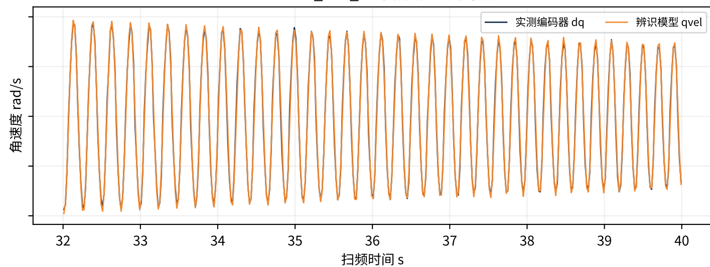
C 组 · R_calf_ · 高频段速度对照
