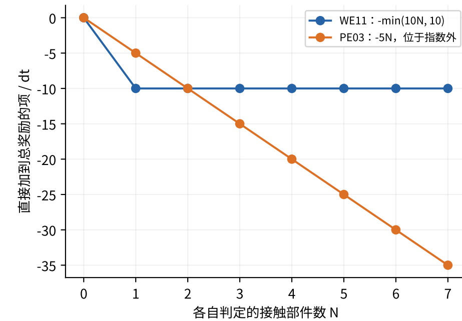
F 碰撞：判定传感量和阈值也不同
