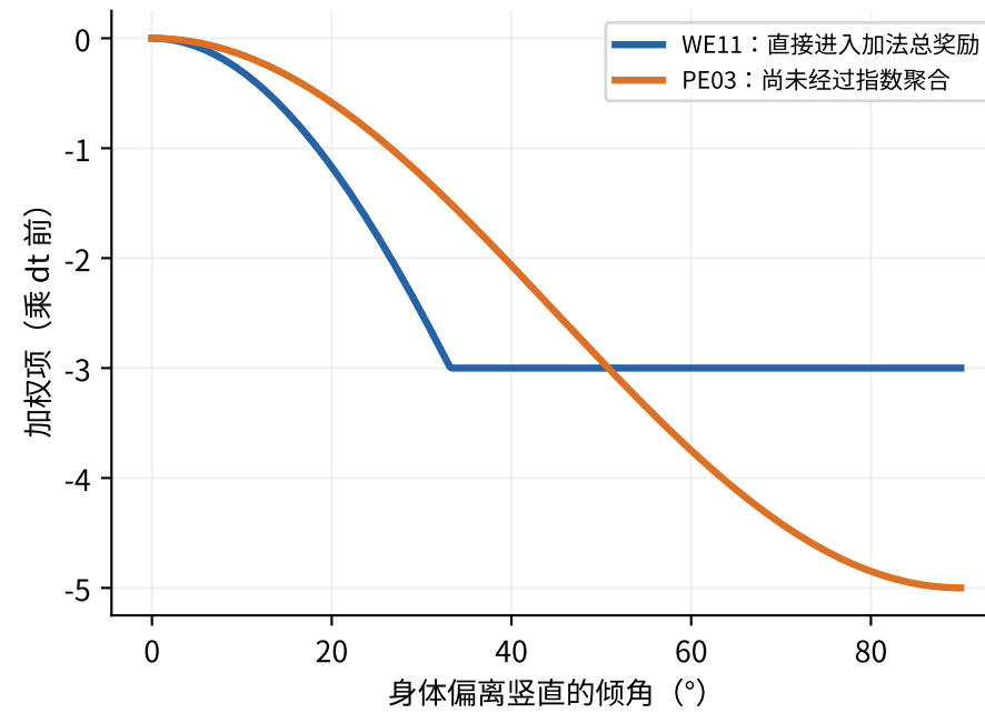
B 姿态：WE11 在约 33.2^\circ 后封顶
