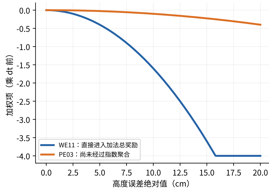
A 高度：WE11 除以 \text{std}^2 ，PE03 不除
