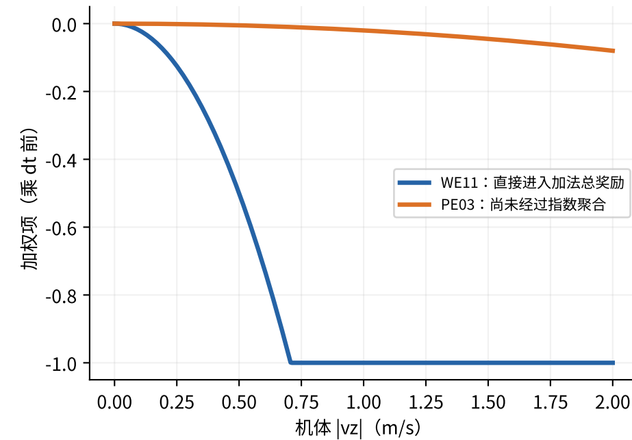
C 竖直速度：当前权重相差 100 倍
