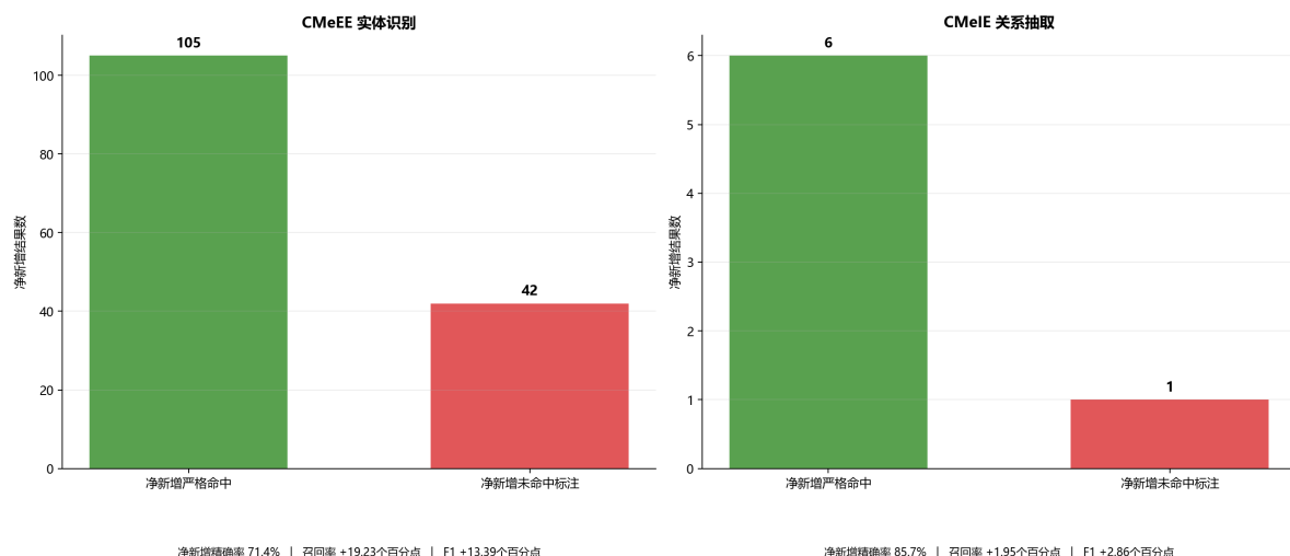
图 7.4 混合方式相对离线方式的净新增结果及严格标注命中情况
