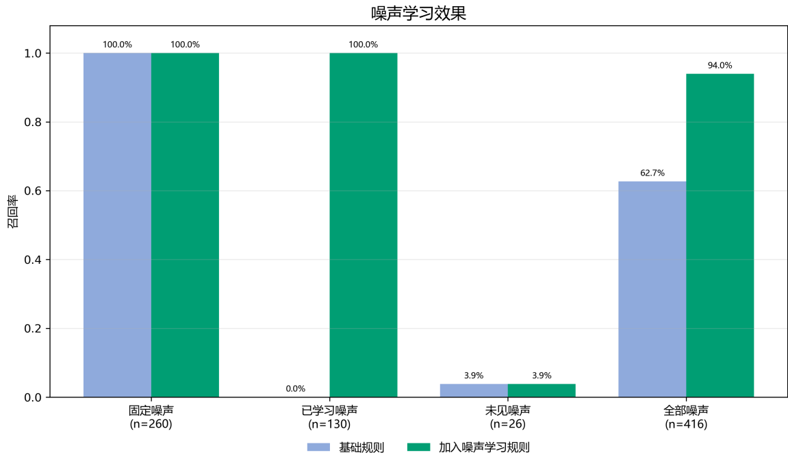
图 7.2 噪声学习前后对比。柱下的 n 表示该类噪声在评测集中的出现次数。
