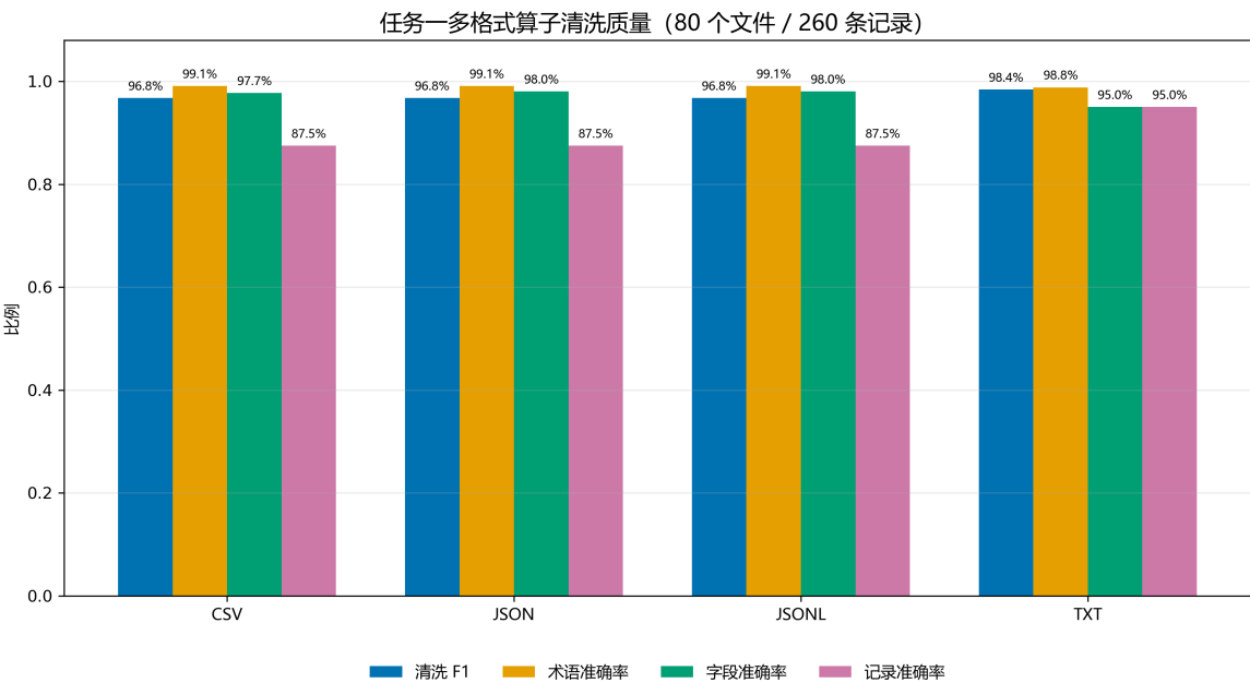
图 7.1 多格式清洗效果。四类链路的清洗 F1 均不低于 96.8%。
