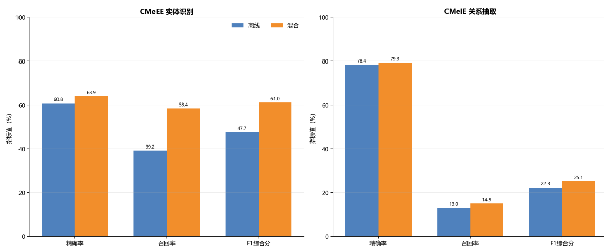
图 7.3 当前同批对比中离线与混合方式的精确率、召回率和 F1
