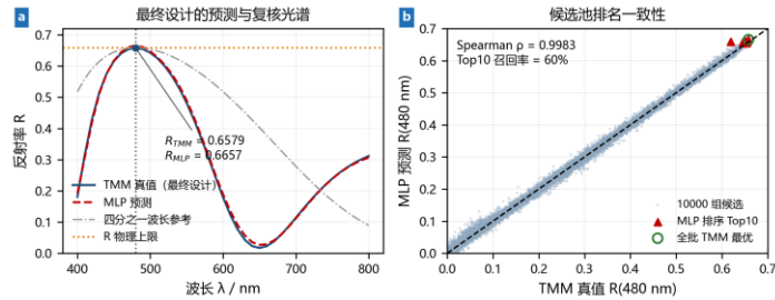
图 7 (a) 最终设计的 MLP 预测光谱与 TMM 复核光谱（标注目标波长与物理上限）；
