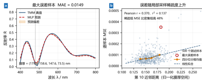
图 8 代表性失败案例：(a) 最大误差样本的 TMM 与 MLP 光谱；(b) 逐样本误差与局部采样密度的关系。
