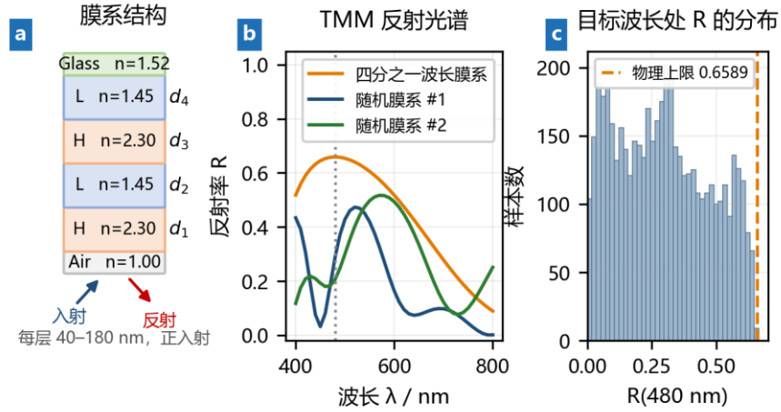
图 2 物理模型与 TMM 数据生成：(a) 膜系结构与折射率（ n_{\sim H} 、 n_{\sim L} 、 n_{\sim s} ）；(b) 三条代表性反射光谱，虚线为 \lambda_{\text{target}} = 480 nm；(c) 5000 组样本在目标波长处的反射率分布，橙色虚线为解析上限。
