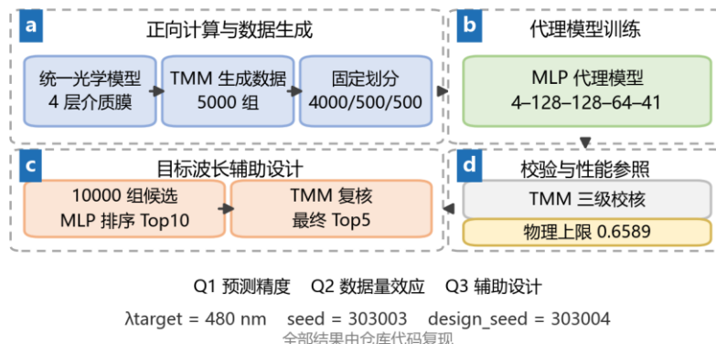
图1 本研究的总体流程：TMM 生成数据、MLP 训练与预测、数据量实验、辅助设计与 TMM 复核。
