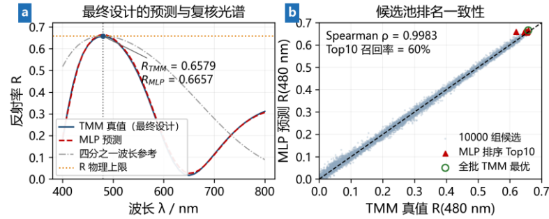
图 7 (a) 最终设计的 MLP 预测光谱与 TMM 复核光谱（标注目标波长与物理上限）；
