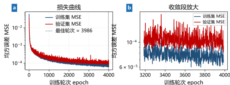
图 4 训练集与验证集的损失曲线。
