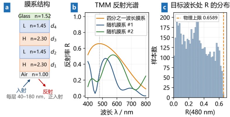
图 2 物理模型与 TMM 数据生成：(a) 膜系结构与折射率 ( n \sim H \sim, n \sim L \sim, n \sim s \sim )；(b) 三条代表性反射光谱，虚线为 \lambda_{\text{target}} = 480 \text{ nm} ；(c) 5000 组样本在目标波长处的反射率分布，橙色虚线为解析上限。
