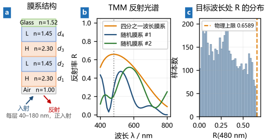
图2 物理模型与 TMM 数据生成：(a) 膜系结构与折射率（ n_H 、 n_L 、 n_s ）；(b) 三条代表性反射光谱，虚线为 \lambda_{\text{target}} = 480 \text{ nm} ；(c) 5000 组样本在目标波长处的反射率分布，橙色虚线为解析上限。
