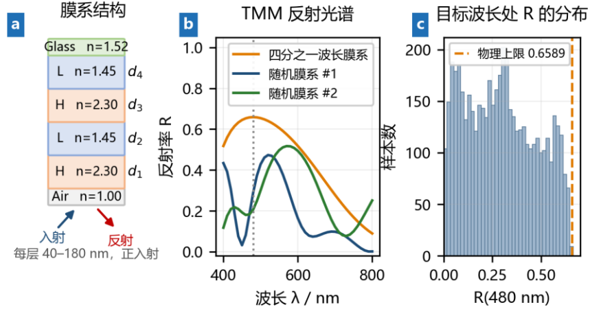
图 2 物理模型与 TMM 数据生成：(a) 膜系结构与折射率（ n_H 、 n_L 、 n_s ）；(b) 三条代表性反射光谱，虚线为 \lambda_{\text{target}} = 480 nm；(c) 5000 组样本在目标波长处的反射率分布，橙色虚线为解析上限。
