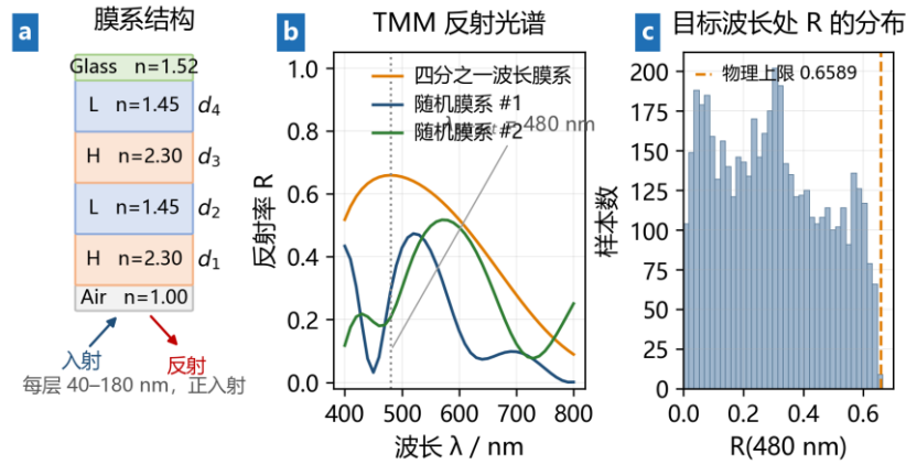
图 2 物理模型与 TMM 数据生成，包括膜系结构、三条代表性反射光谱与 5000 组样本在目标波长处的反射率分布。
