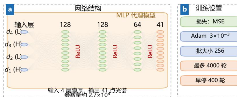
图3 MLP 代理模型结构：输入 4 层膜厚，经 128–128–64 三个隐藏层，输出 41 点反射率。
