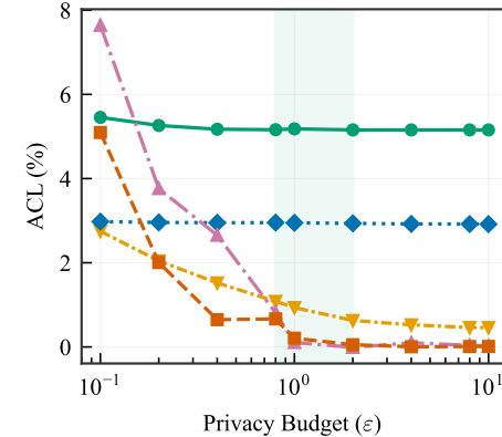
Diabetes ( N=70,692 , F=21 )
