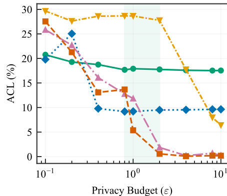
Diabetes ( N=70,692 , F=21 )
