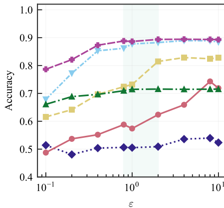
GNB
