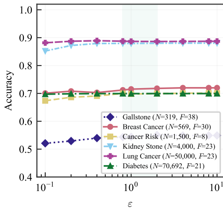
SVM
