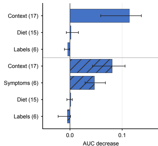
d Random forest / AUC
