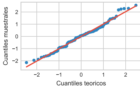
Q-Q Normal
