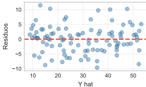
Residuos vs Ajustados
