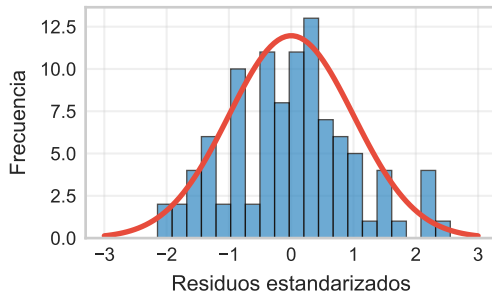
Histograma Residuos
