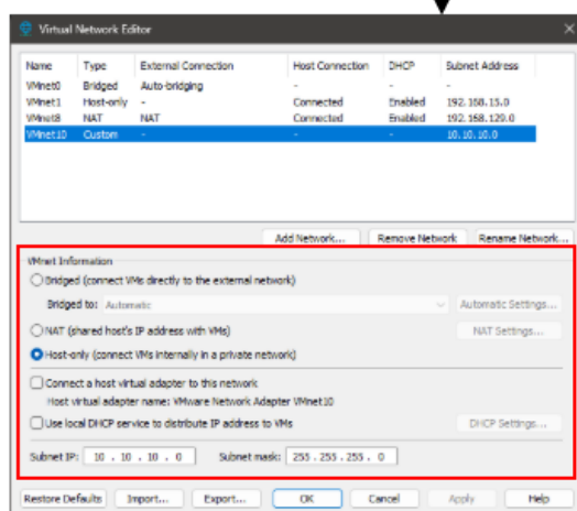
Figura 14 Configuración de la red interna VMnet10 en VMware Workstation.
