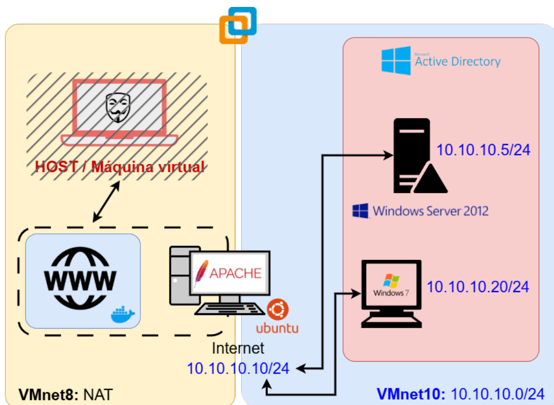
Figura 6 Diagrama completo de la infraestructura del laboratorio, mostrando los sistemas, servicios, segmentos de red y relaciones entre componentes.
