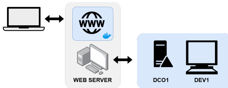
Figura 11 Diagrama de la arquitectura lógica del laboratorio, mostrando los niveles de acceso y las relaciones entre los distintos sistemas.
