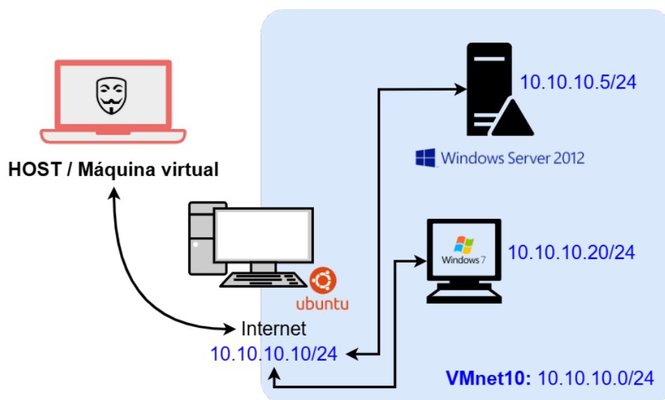
Figura 12 Esquema detallado de la segmentación de red y configuración de interfaces en VMware Workstation.
