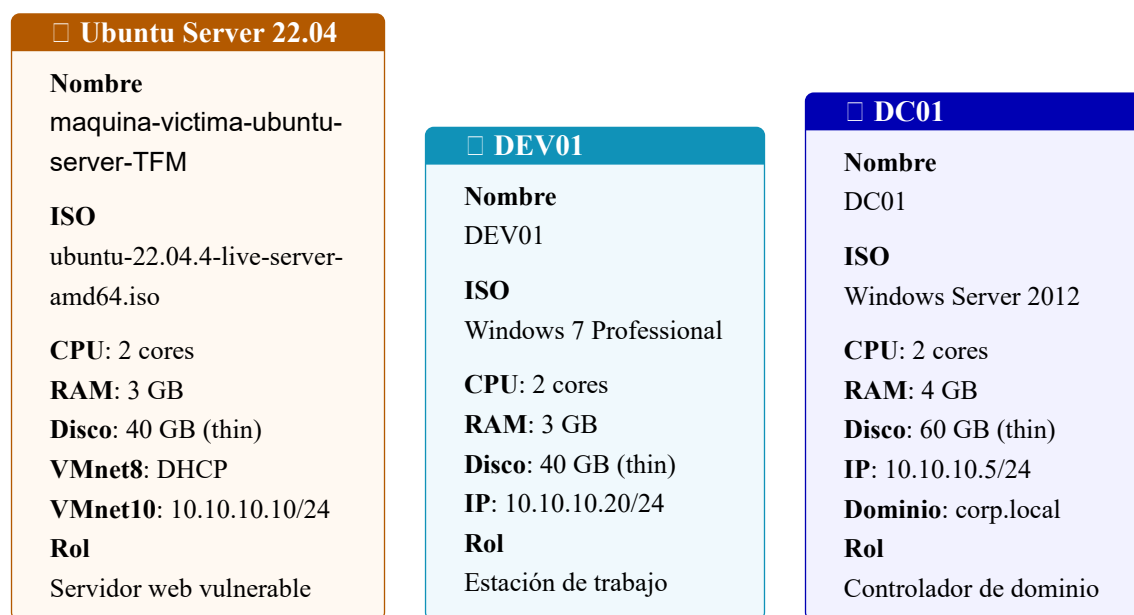
Figura 9 Configuración de las máquinas virtuales que componen la infraestructura del laboratorio.
