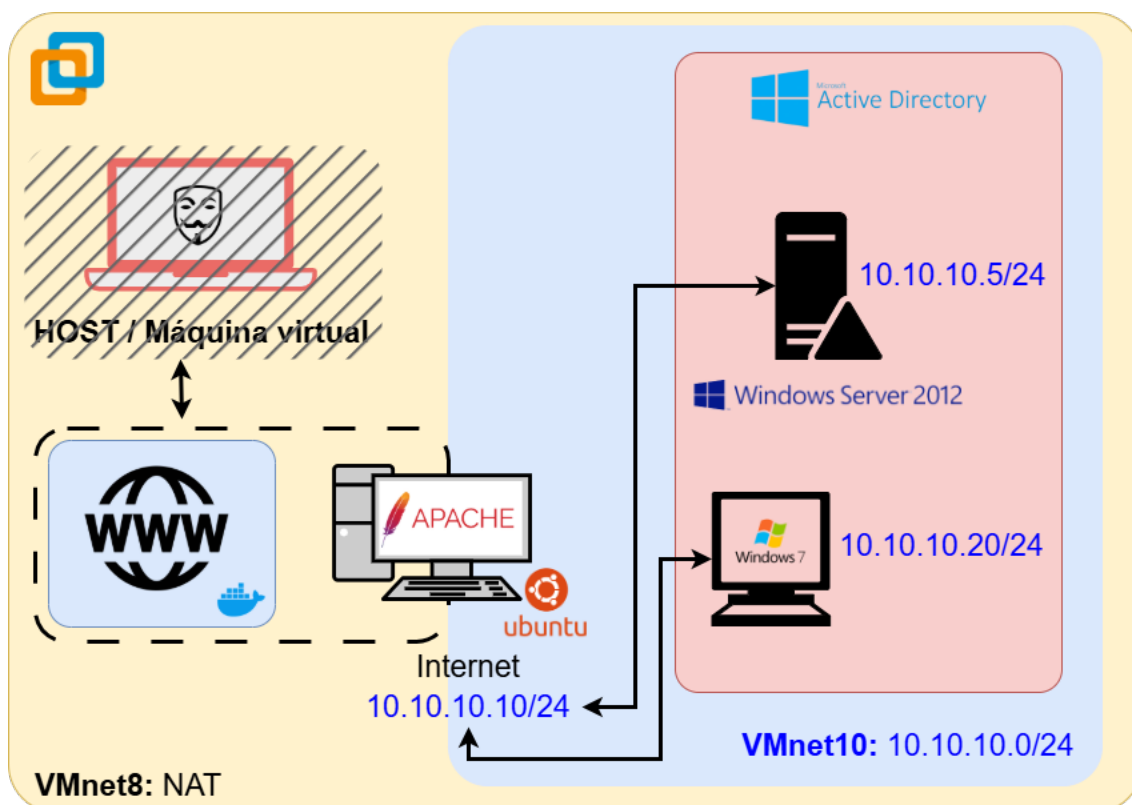
Figura 8 Diagrama completo de la infraestructura del laboratorio, mostrando los sistemas, servicios, segmentos de red y relaciones entre componentes.
