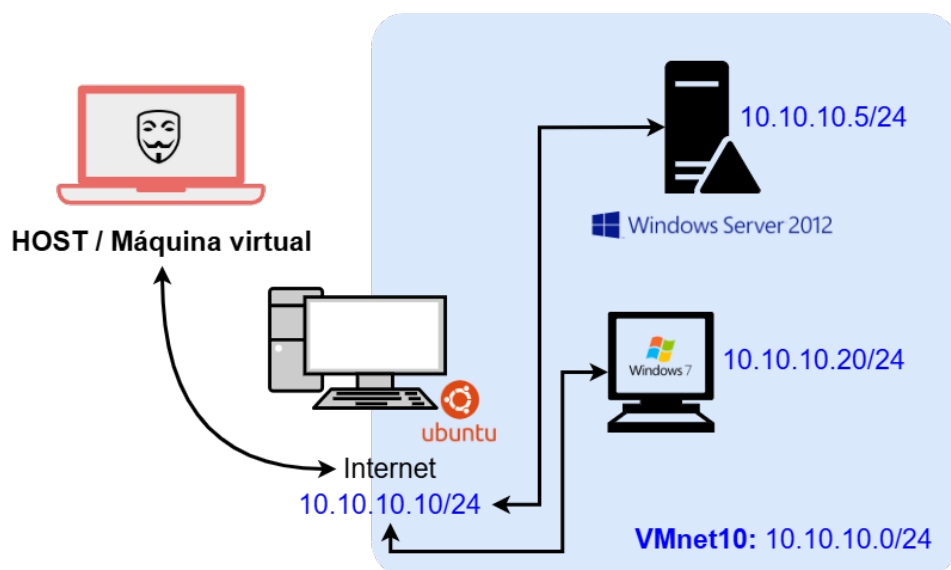
Figura 13 Esquema detallado de la segmentación de red y configuración de interfaces en VMware Workstation.
