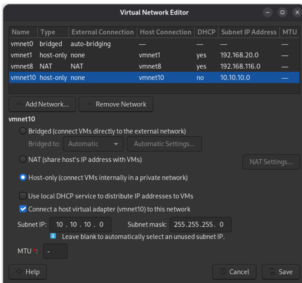
Figura 14 Configuración de la red en VMware
