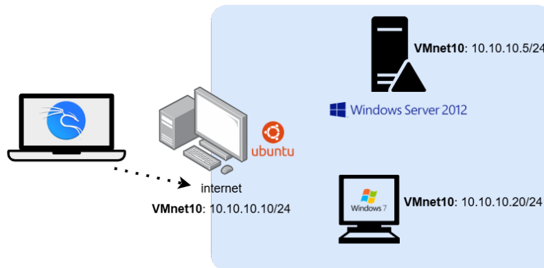
Figura 11 Esquema detallado de la segmentación de red y configuración de interfaces en VMware Workstation.
