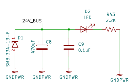
24V Bus
