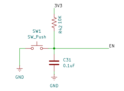
Button for EN pin
