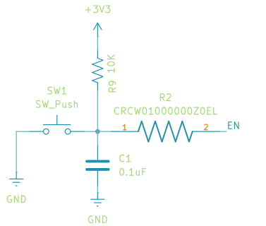
Button for EN pin
