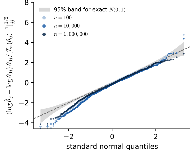
(d) normal Q-Q, \log \sigma^2
