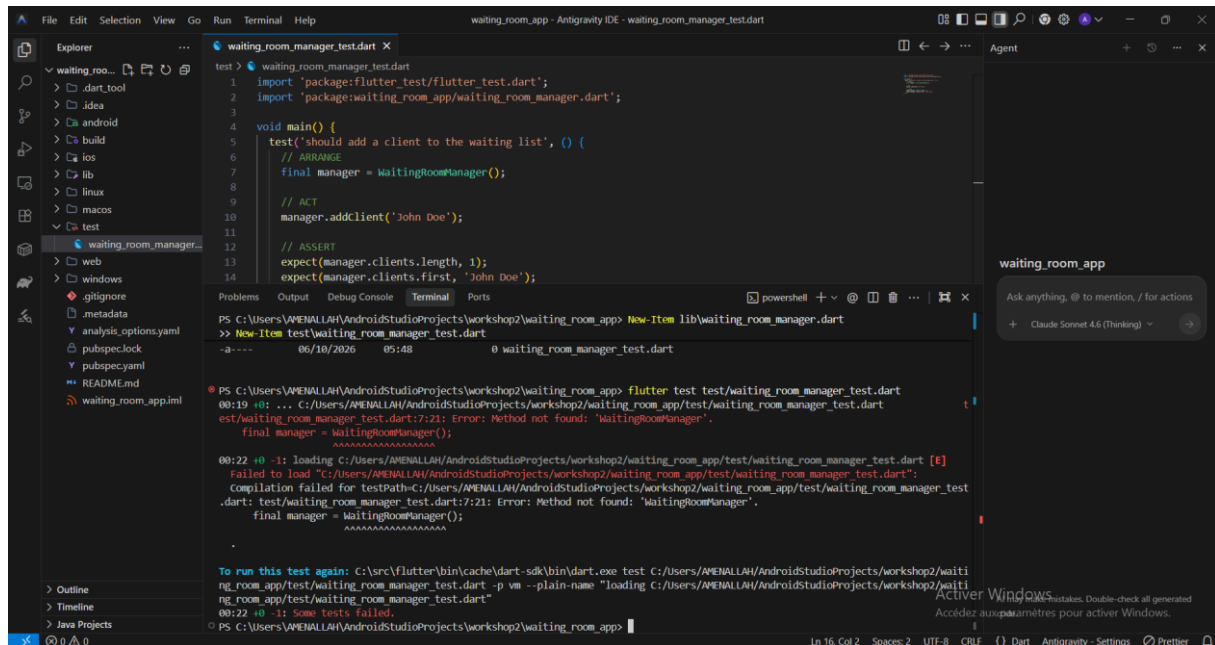
Figure 1 : Test unitaire d'ajout en échec
