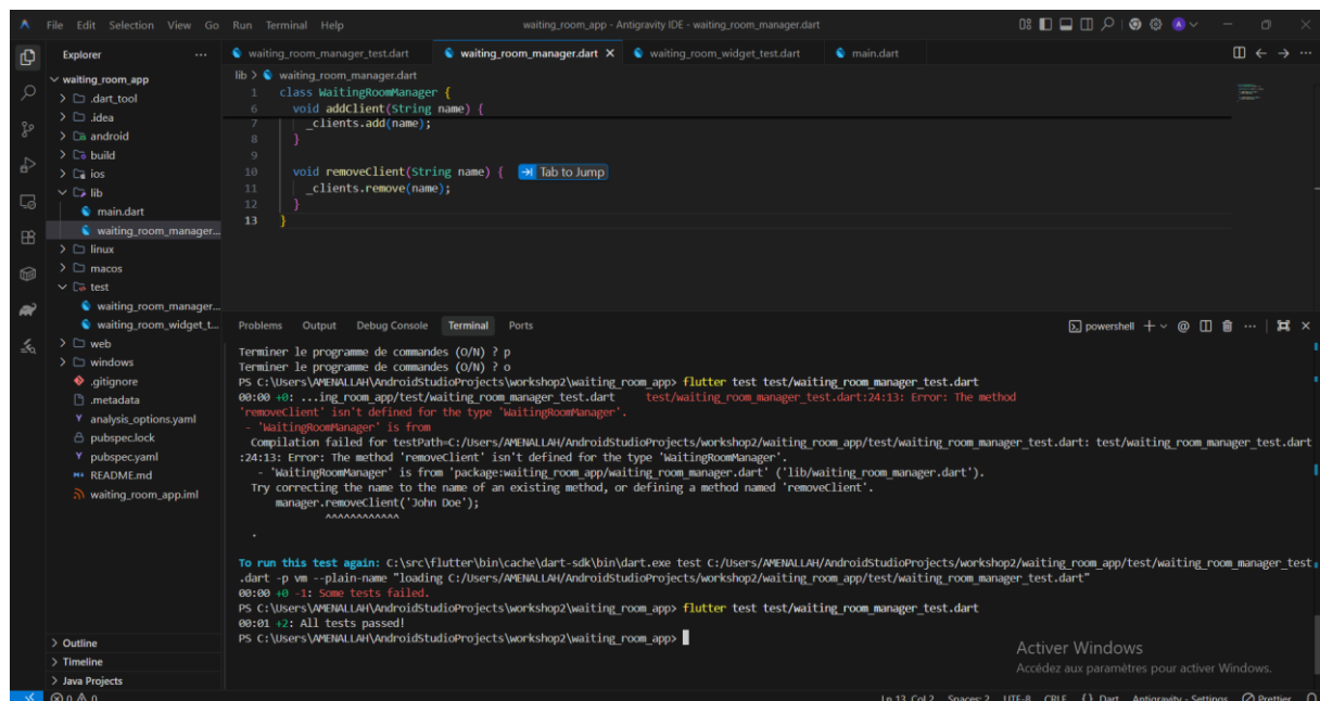
Figure 4 : Fonction de suppression, test unitaire rouge puis vert
