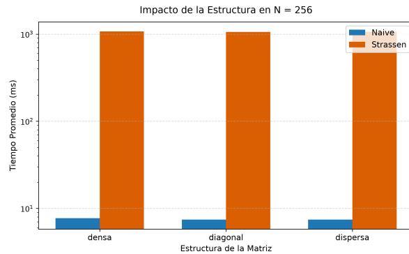
Figura 8: Estructura interna.
