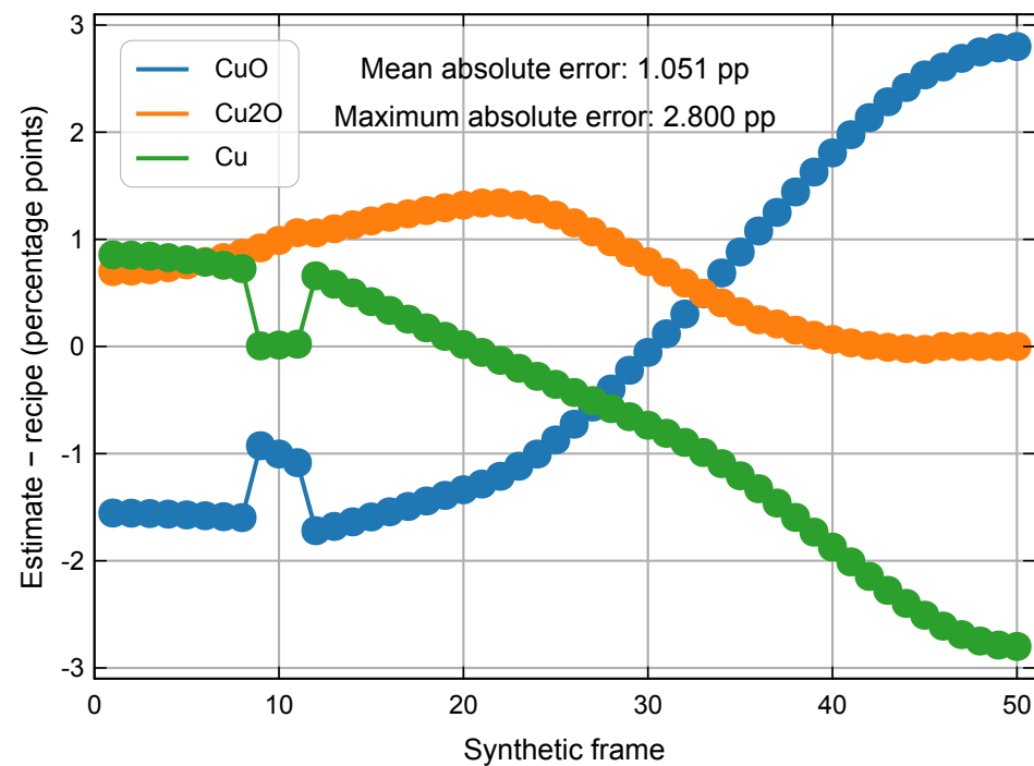
c MCR-ALS error
