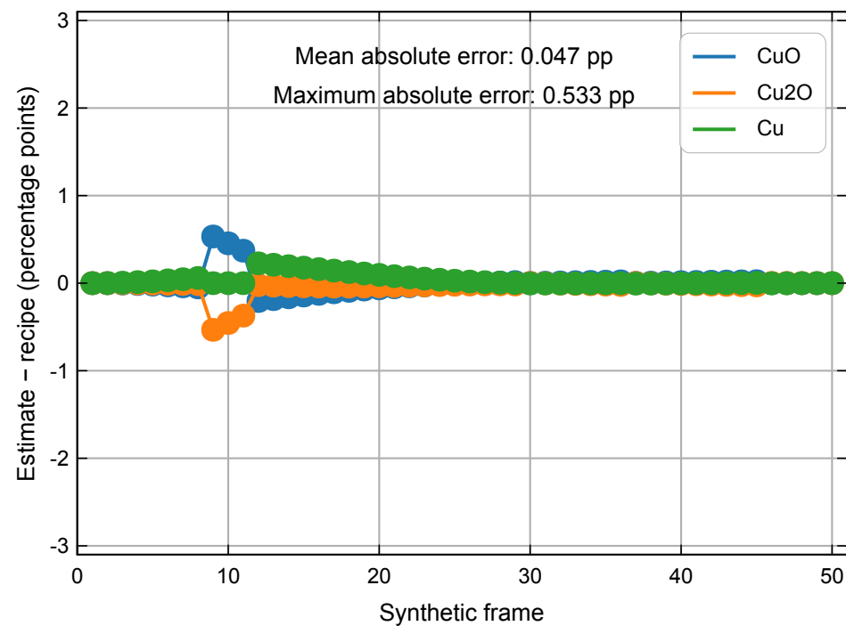
d LCF error
