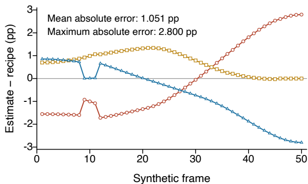
c MCR-ALS error
