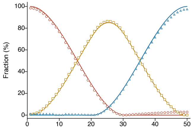
a MCR-ALS (blind)
