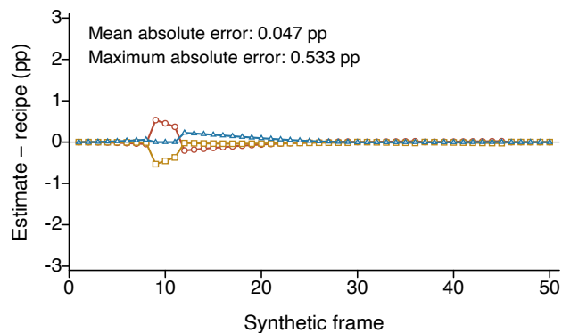
d LCF error
