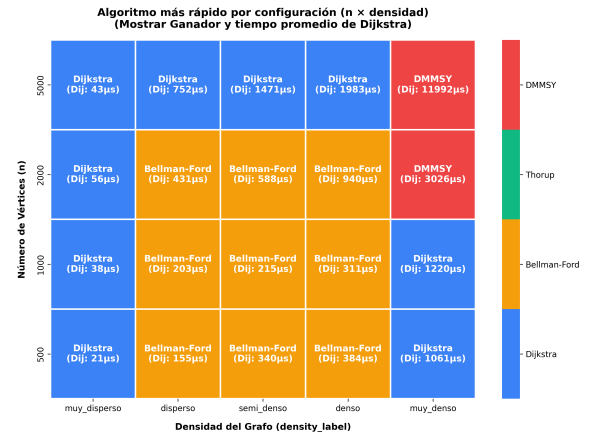
Figura 4. Algoritmo ganador en tiempo promedio por configuración. Azul representa a Dijkstra, naranja a Bellman-Ford y rojo a DMMSY.
