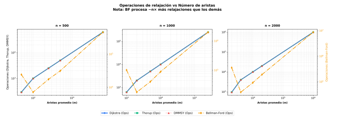
Figura 3. Operaciones de relajación vs. m en escala doblemente logarítmica. Las curvas de Dijkstra, Thorup y DMMSY coinciden de manera idéntica al explorar en orden de distancias. Bellman-Ford requiere un volumen mayor.
