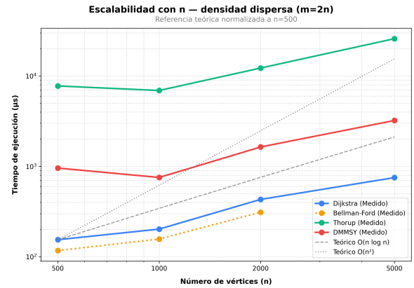
Figura 5. Escalabilidad en tiempo frente a n para m = 2n . Las líneas punteadas muestran las referencias teóricas asíntóticas normalizadas al punto inicial.
