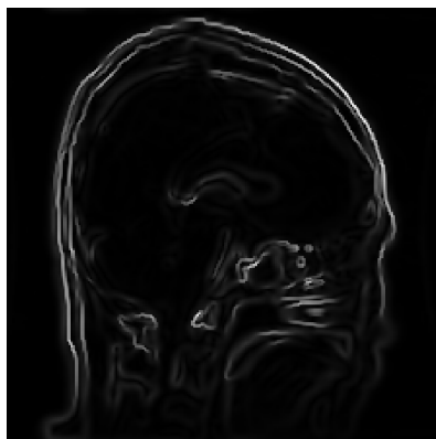
Énergie directionnelle
