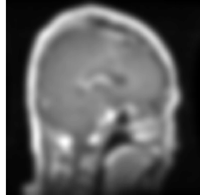
Basse fréquence
