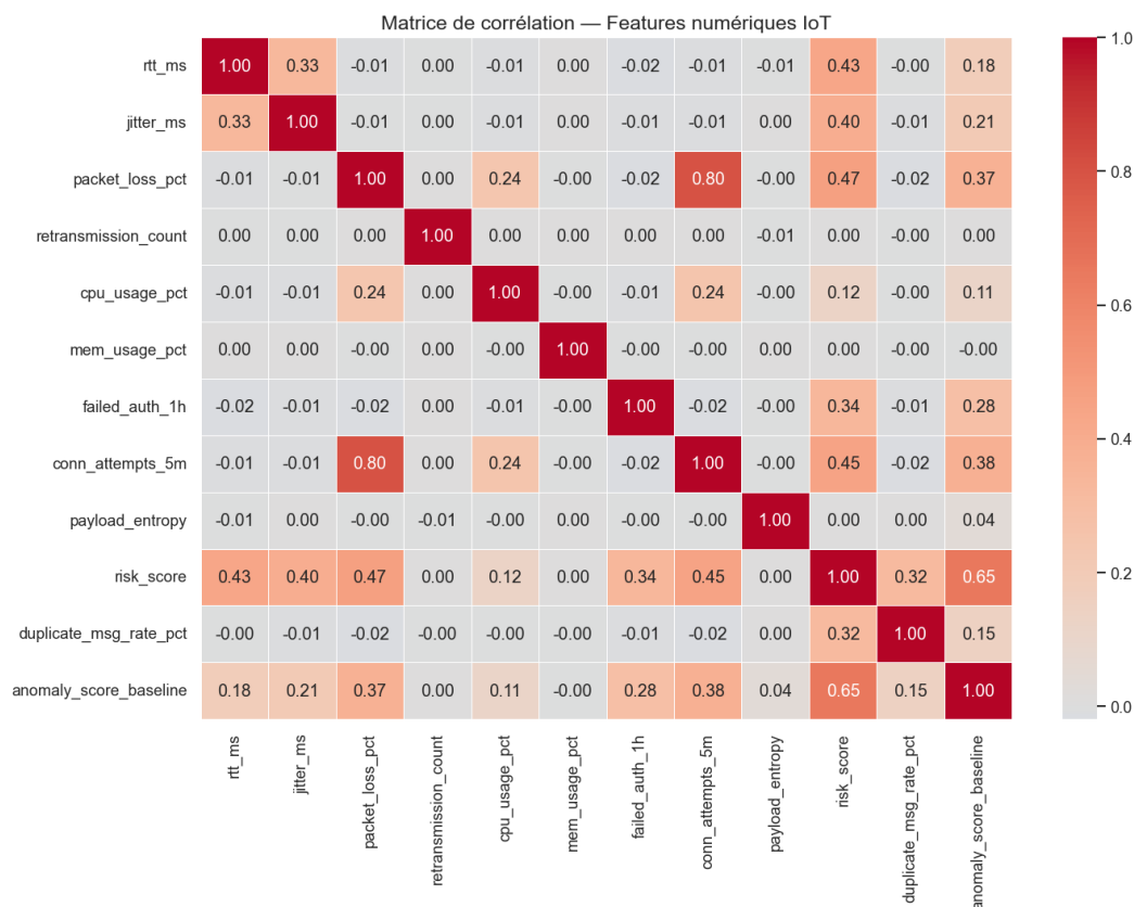
Fig. 4.21 : Analyse exploratoire — matrice de corrélation des features numériques
