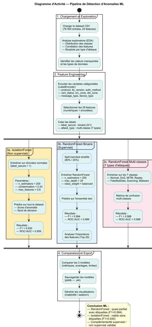
Fig. 4.17 : Pipeline d'apprentissage automatique (collecte, features, entraînement, évaluation, SIEM)
