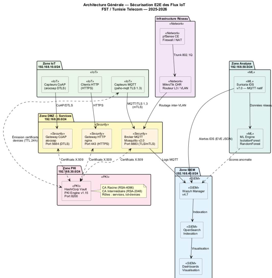
Fig. 1.3 : Vue d'ensemble de l'architecture de sécurisation proposée
