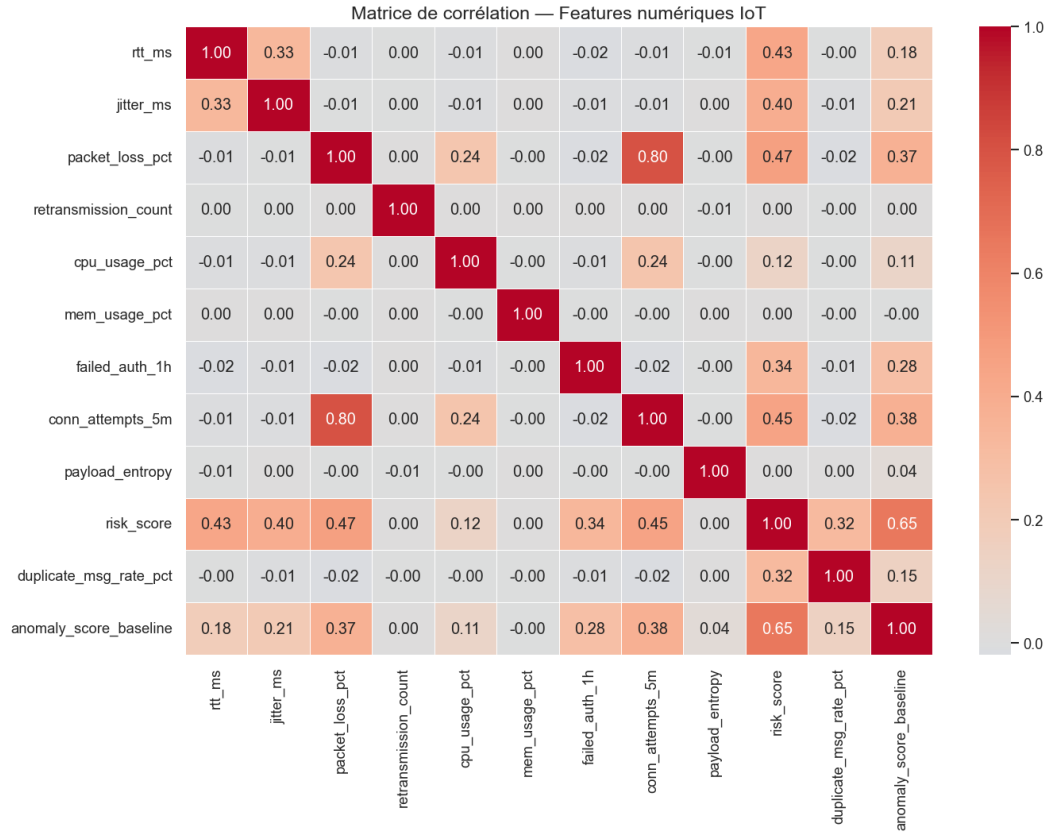
Fig. 4.17 : Analyse exploratoire — matrice de corrélation des features numériques
