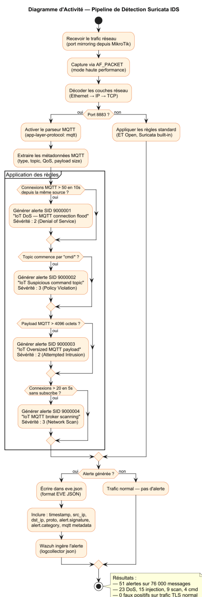
Fig. 4.14 : Chaîne de détection Suricata → Wazuh (IDS+SIEM)
