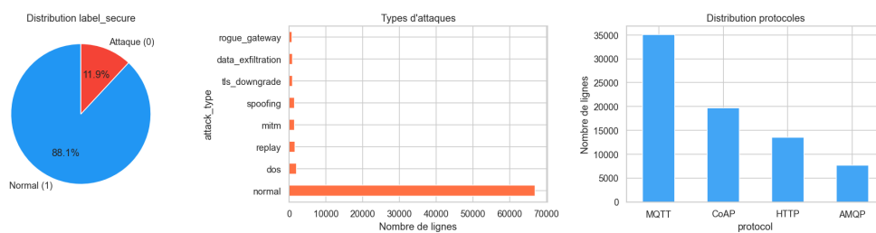
Fig. 4.16 : Analyse exploratoire — distribution des classes
