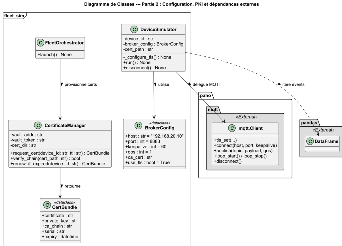
Fig. 3.6 : Diagramme de classes — Partie 2 : configuration, PKI et dépendances externes ( BrokerConfig , CertificateManager , CertBundle )
