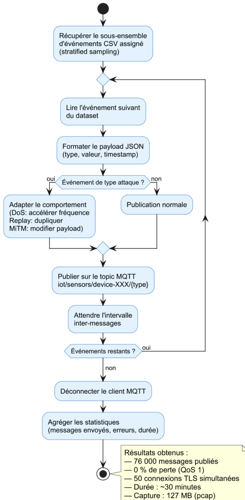
Fig. 3.7 : Activité — Phase 3 : boucle de publication MQTT et agrégation des résultats
