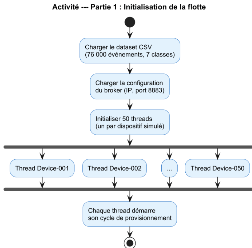
Fig. 3.5 : Activité — Phase 1 : initialisation des 50 threads de la flotte
