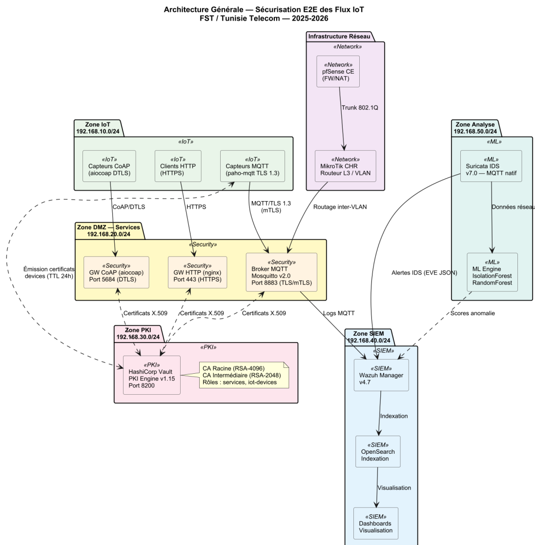
Fig. 4.1 : Architecture globale en défense en profondeur
