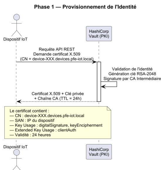
Fig. 4.5 : Flux E2E — Phase 1 : provisionnement de l’identité
