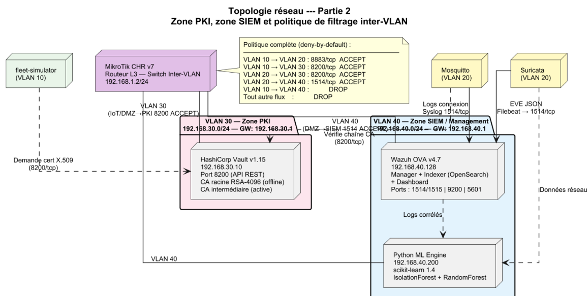
Fig. 4.4 : Topologie réseau — Partie 2 : zone PKI (VLAN 30), zone SIEM/Analyse (VLAN 40) et politique de filtrage inter-VLAN complète
