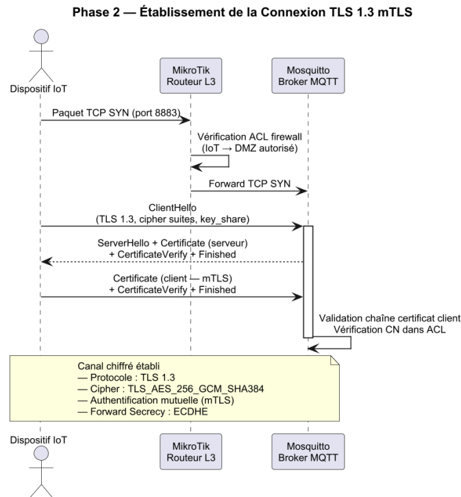
Fig. 4.6 : Flux E2E — Phase 2 : établissement de la connexion TLS 1.3 mTLS
