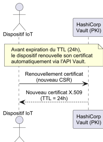
Fig. 4.9 : Flux E2E — Phase 5 : rotation automatique des certificats
