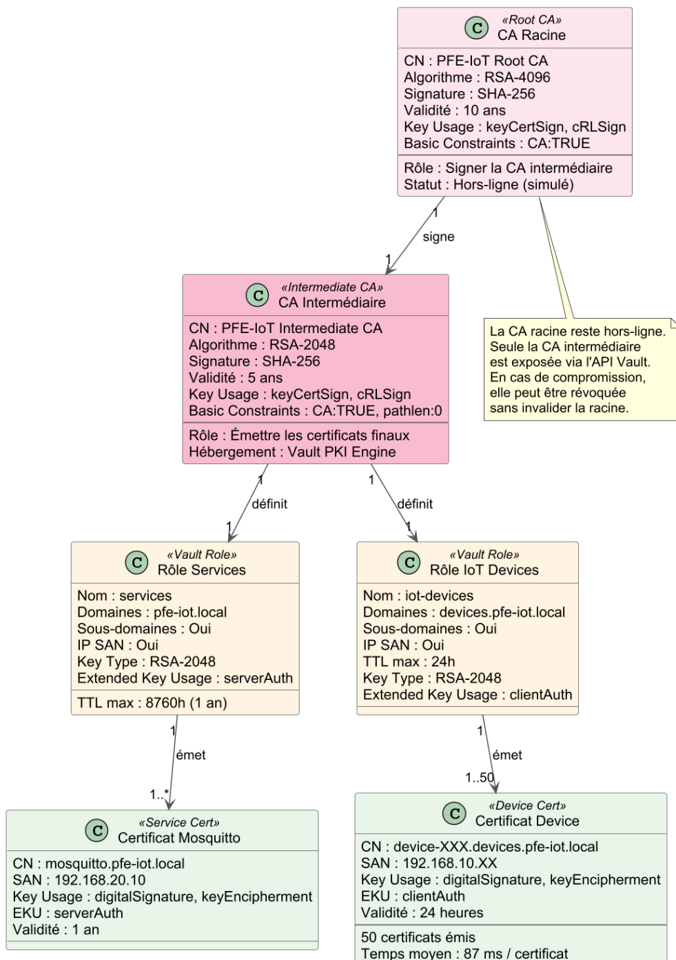
Fig. 4.10 : Hiérarchie de la PKI à deux niveaux (CA racine offline + CA intermédiaire Vault)
