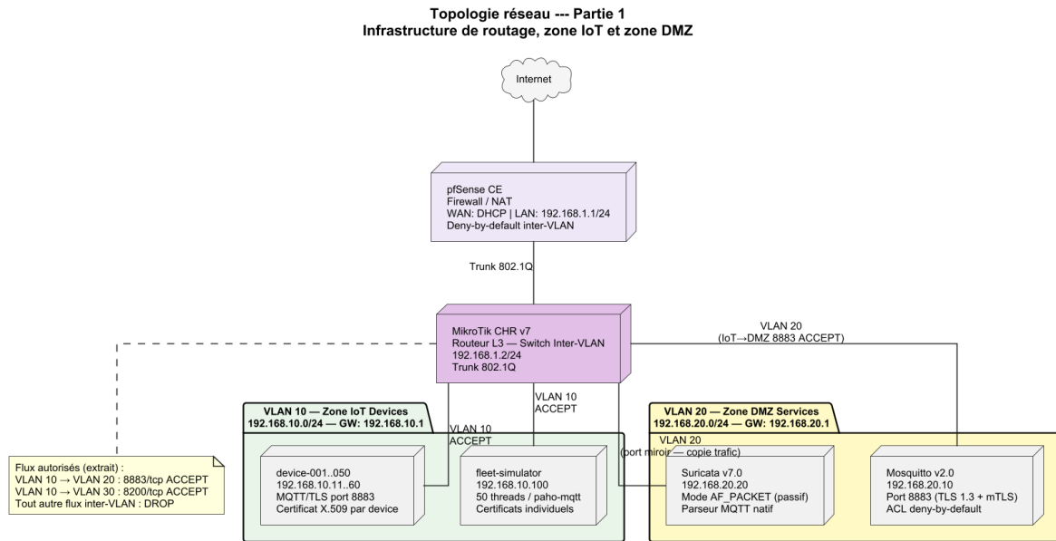
Fig. 4.3 : Topologie réseau — Partie 1 : infrastructure de routage (pfSense, MikroTik), zone IoT (VLAN 10) et zone DMZ (VLAN 20)
