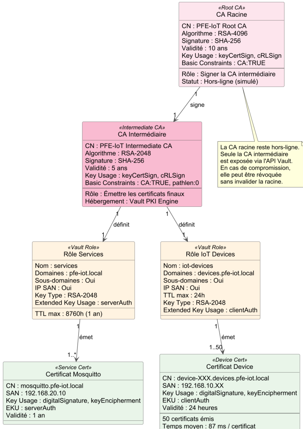
Fig. 4.12 : Hiérarchie de la PKI à deux niveaux (CA racine offline + CA intermédiaire Vault)
