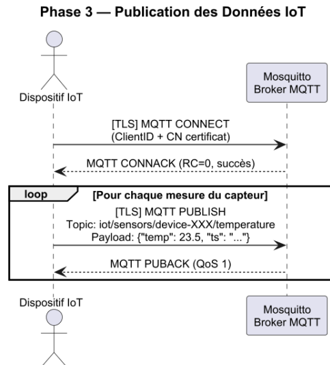
Fig. 4.9 : Flux E2E — Phase 3 : publication des données IoT
