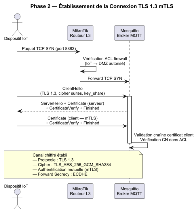
Fig. 4.8 : Flux E2E — Phase 2 : établissement de la connexion TLS 1.3 mTLS
