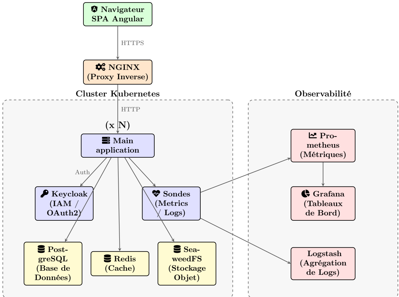
Figure 3 – Diagramme de Déploiement de l'Infrastructure ResiAIAC
