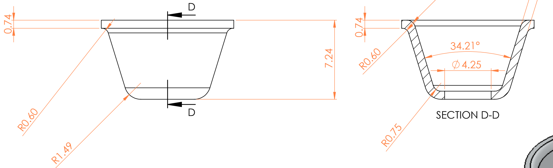
Part3_Pad1
