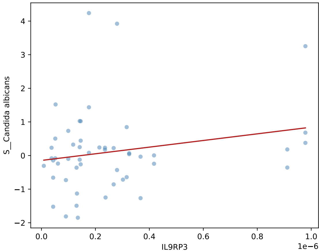
IL9RP3 vs. Candida albicans (+-4w, CD, n=50)
