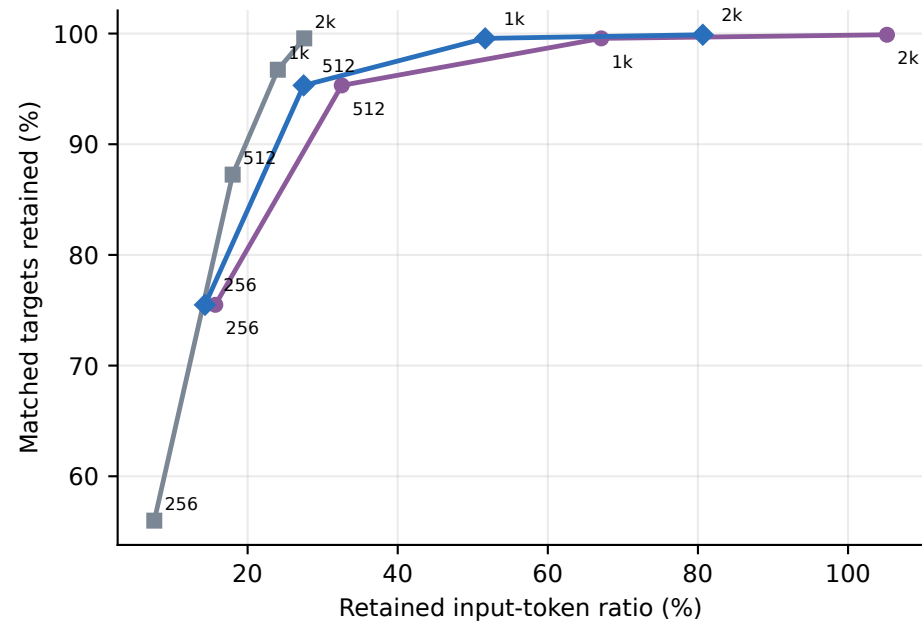
ToolACE
