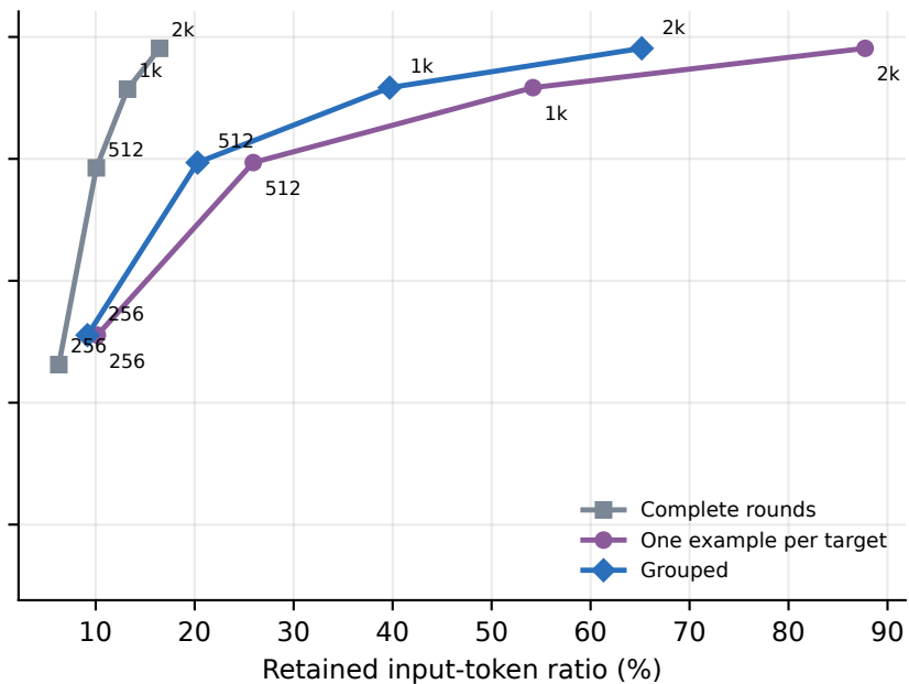
ReTool
