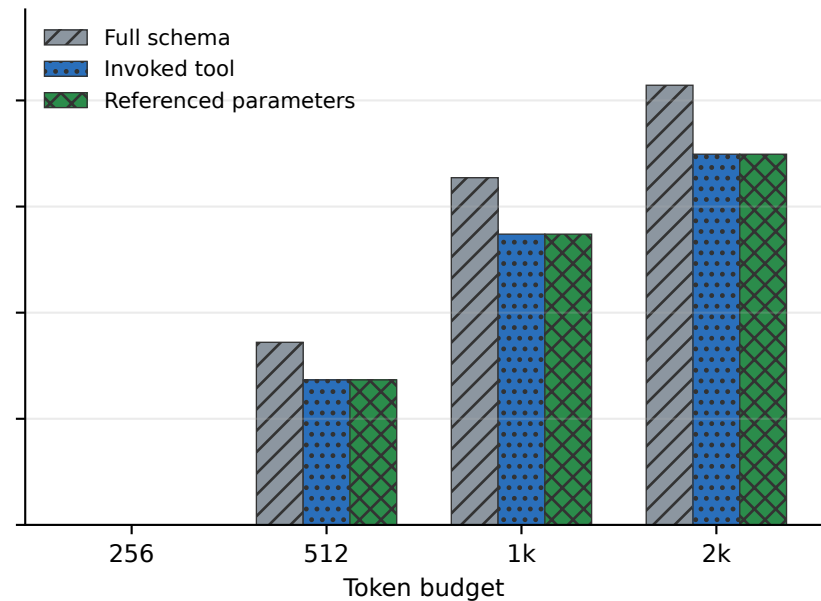
ReTool
