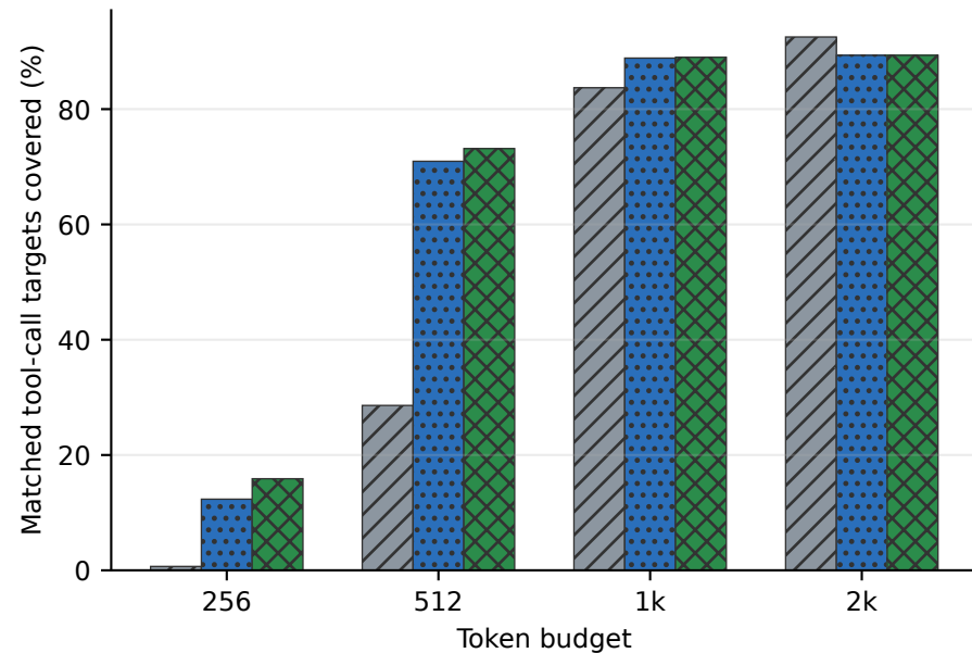
ToolACE
