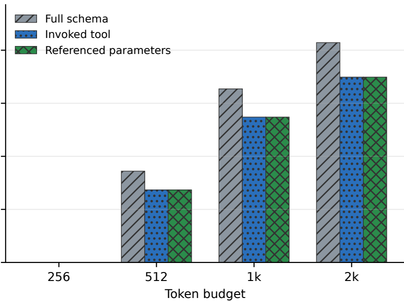
(b) ReTool
