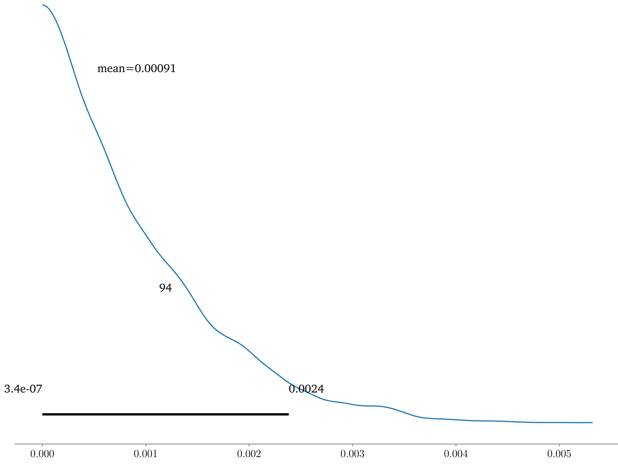
beta_bias
