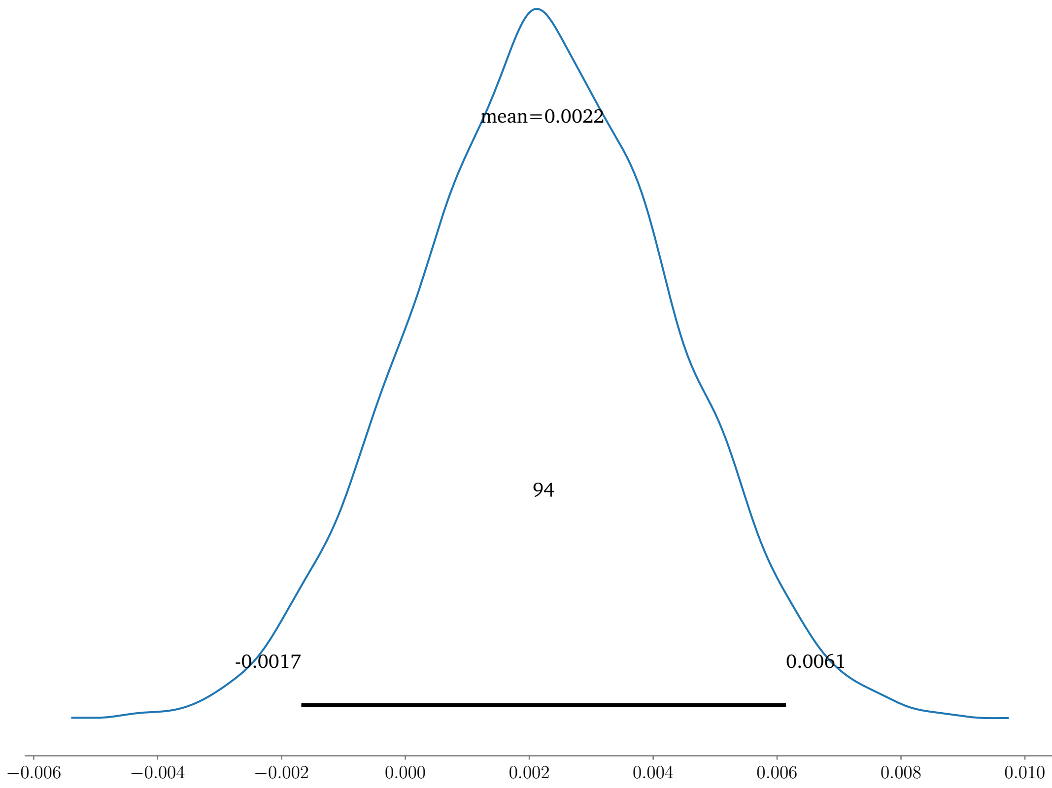
beta_bias
