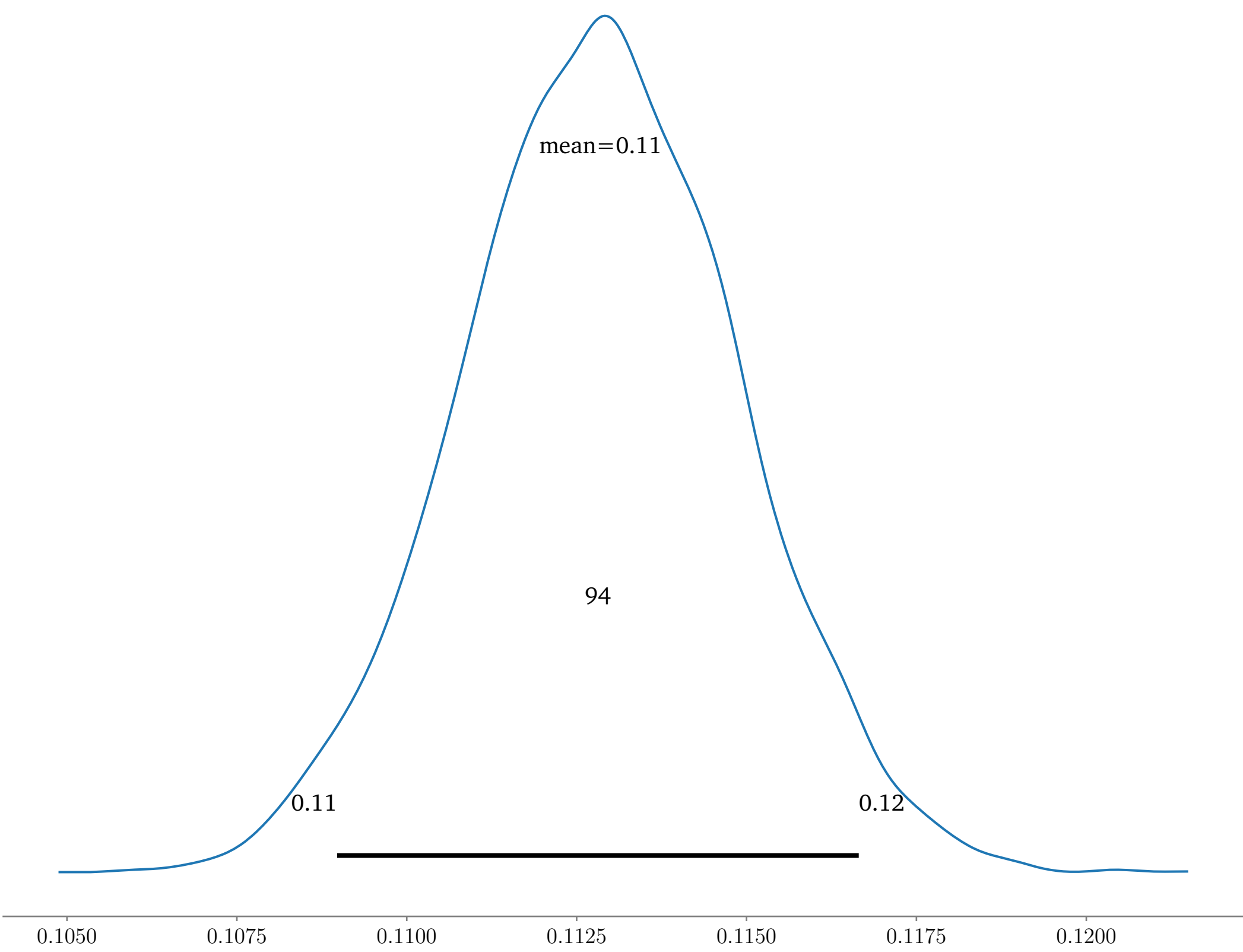
beta_sampler
