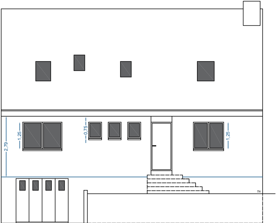
FACADE EST
