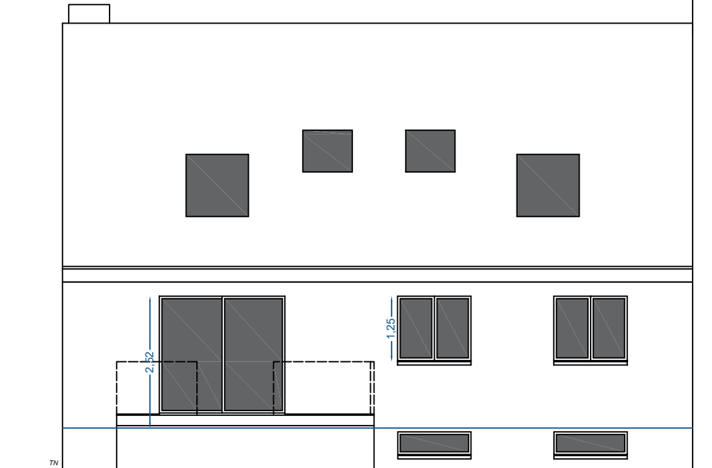
FACADE OUEST
