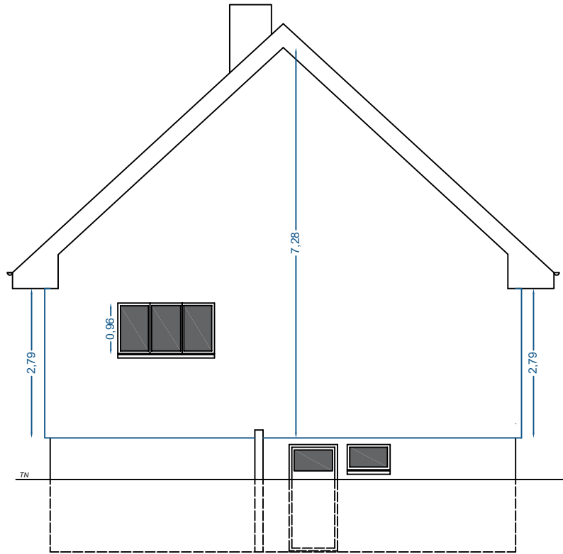
FACADE NORD
