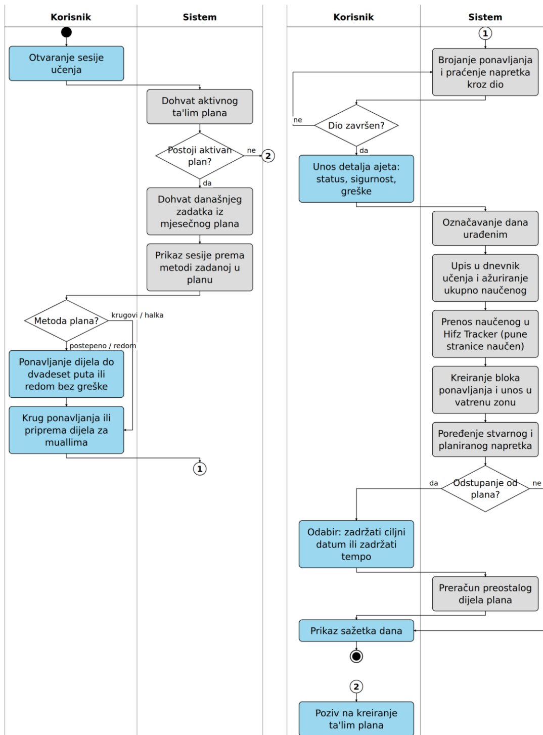
Slika 16. Dijagram aktivnosti, izvršavanje dnevnog učenja
