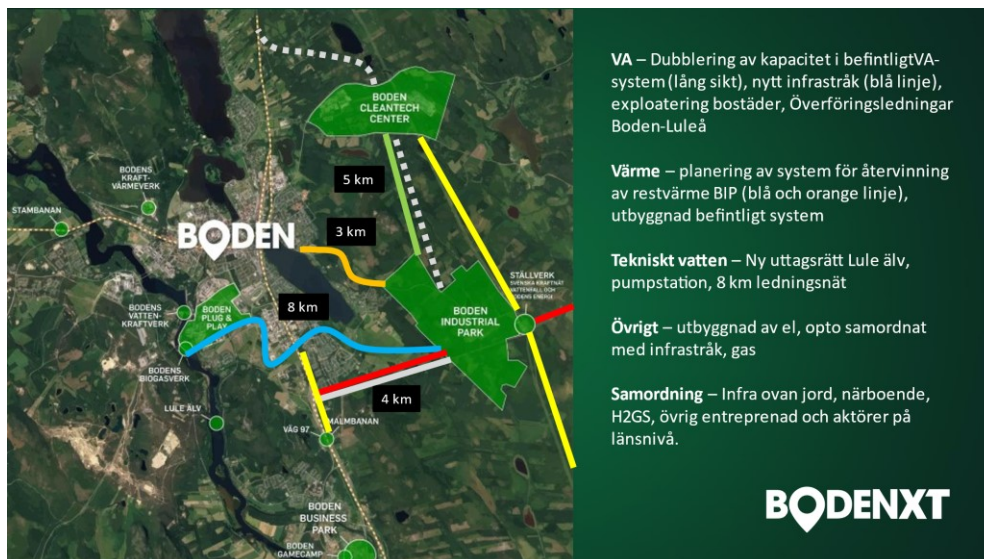
Bild 2 - Översiktlig beskrivning av planerad sträckning av tekniskt vatten och vatten- och avlopp.
