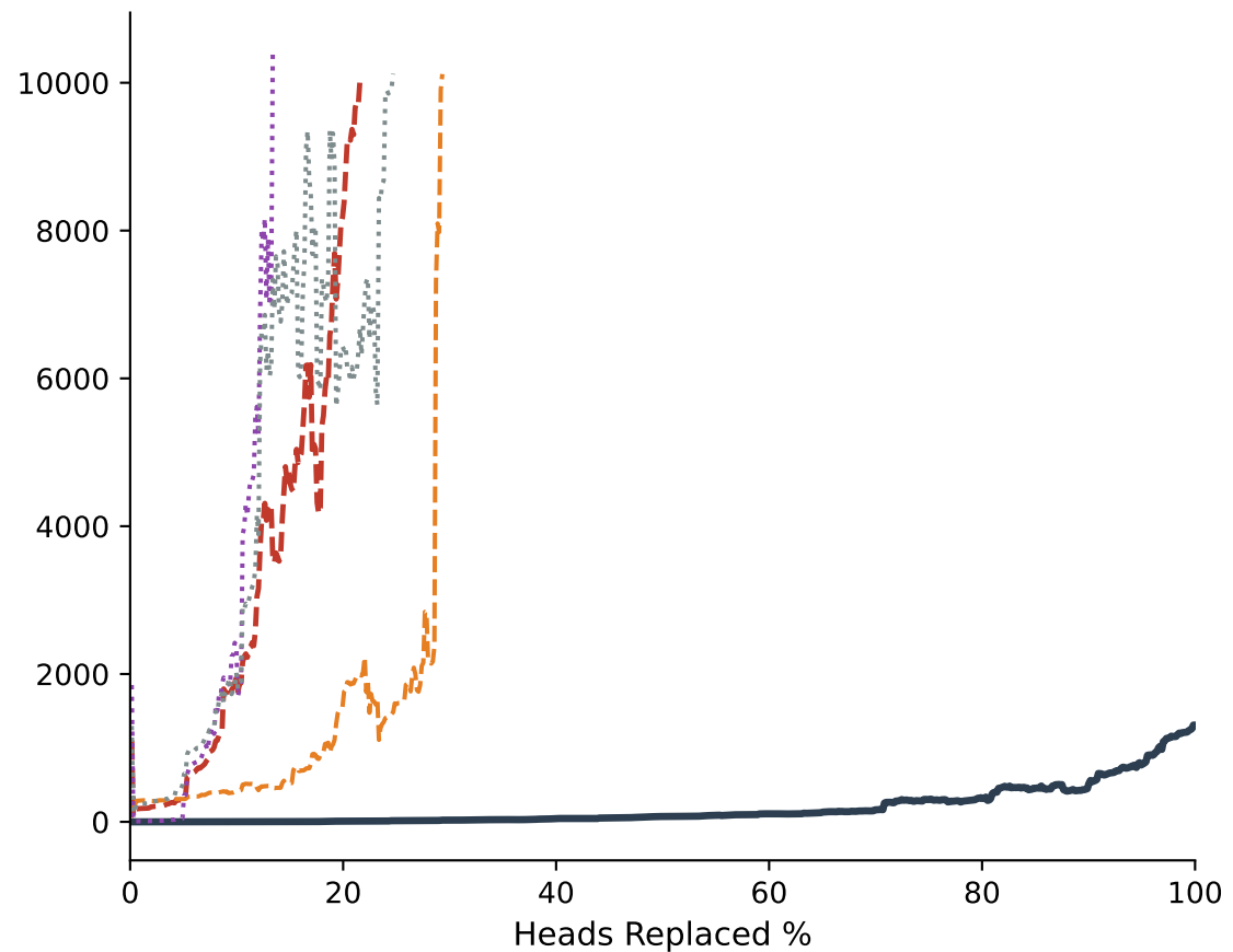
Llama-3.2-3B
