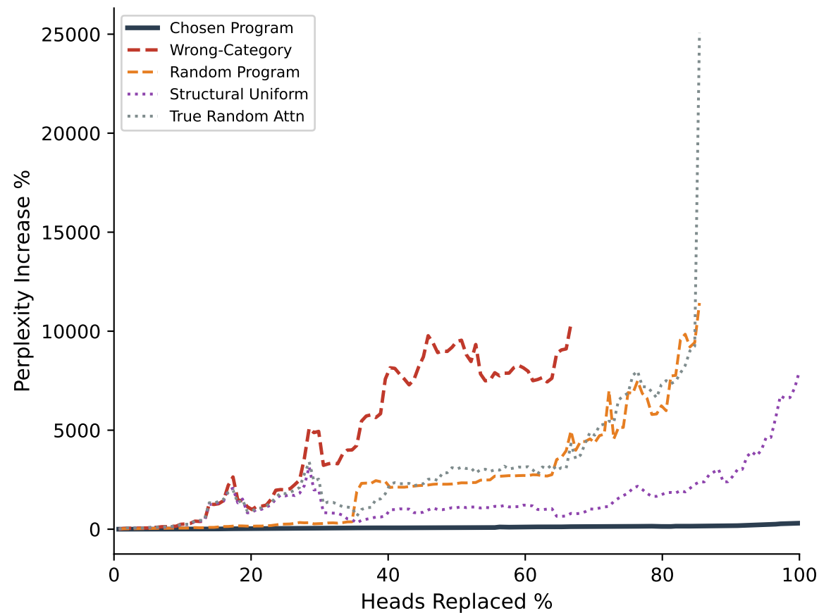
GPT-2
