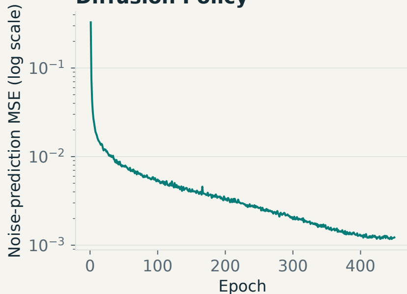
Diffusion Policy
