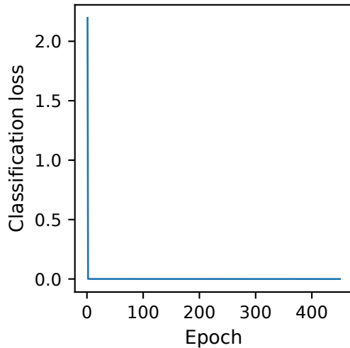
(b) IBC
