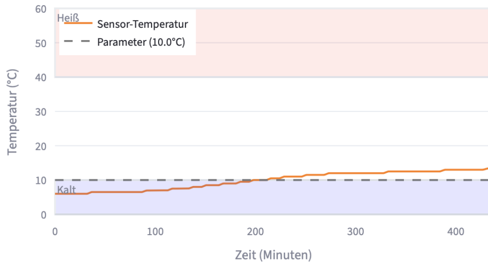
Abbildung 4.11. Temperaturverlauf während Ladesitzung B (9,8 °C Mittelwert): Die Batterietemperatur steigt über 450 min von 6 °C auf 14 °C. Die farbigen Zonen markieren den kalten (< 10 °C, blau) und heißen (> 40 °C, rot) Bereich. Die gestrichelte Linie zeigt den eingestellten Temperaturparameter von 10 °C (Daten aus eigener Messung, Screenshot aus der Softwareanwendung)
