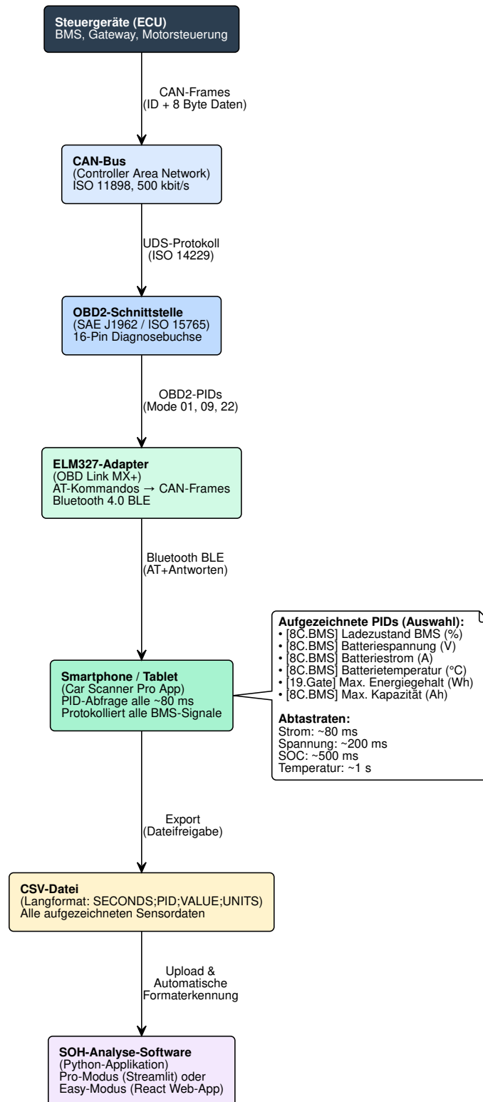
Abbildung 2.6. OB2-Kommunikationskette: Vom Steuergerät über den CAN-Bus und die OB2-II-Schnittstelle bis zur Datenaufzeichnung und Analyse. Die angegebenen Abtastraten wurden aus eigenen Messdaten bestimmt (eigene Darstellung).
