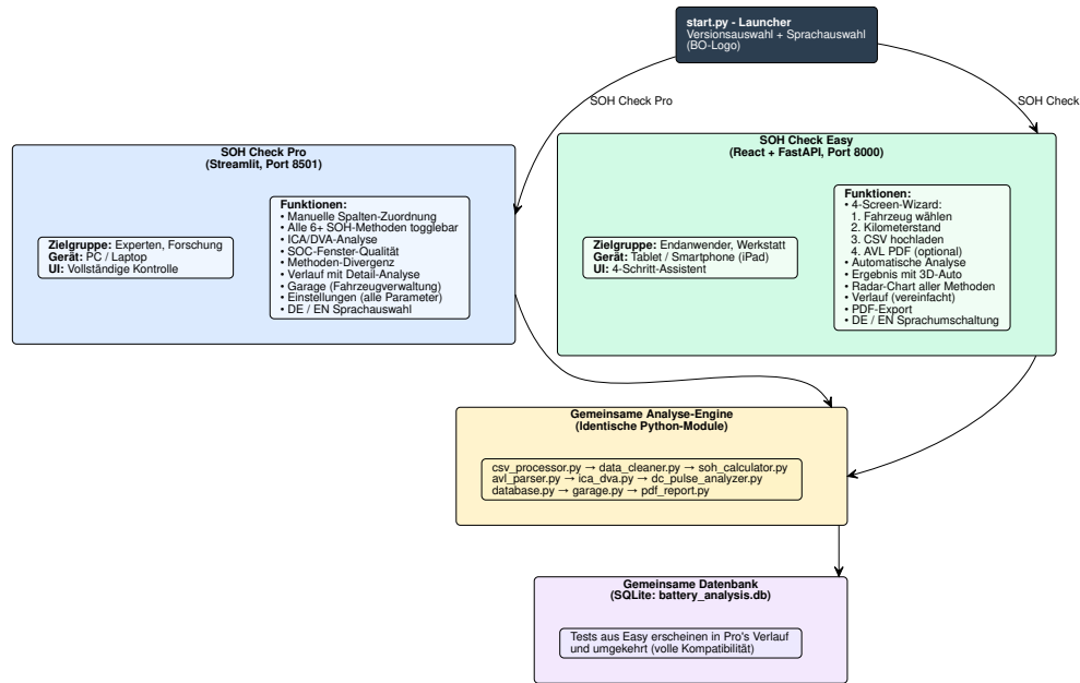
Abbildung 3.14. Architekturvergleich der beiden Betriebsmodi: Pro-Modus (Streamlit, für Experten) und Easy-Modus (React + FastAPI, für Endanwender) mit gemeinsamem Analysekernel und geteilter Datenbank (eigene Darstellung)
