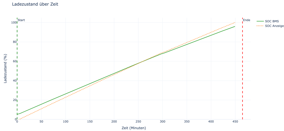
Abbildung 4.3. SOC-Verlauf einer vollständigen AC-Wallbox-Ladung des VW ID.4 (Ladesitzung A, 19°C): SOC_{BMS} (grün) und SOC_{Anzeige} (orange) über die Ladedauer von 465 min (Daten aus eigener Messung)
