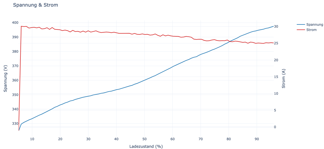
Abbildung 4.12. Spannung und Strom über den SOC-Verlauf (Ladesitzung A, 19 °C): In der CC-Phase steigt die Packspannung von \approx 330 V auf \approx 397 V bei annähernd konstantem Ladestrom von \approx 30 A (Daten aus eigener Messung, Diagramm aus der Softwareanwendung)
