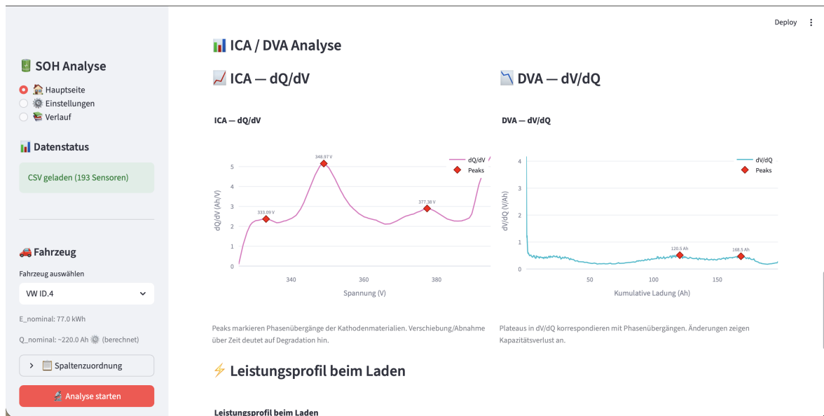
Abbildung 4.17. ICA-Kurve ( dQ/dV vs. Spannung) des VW ID.4 während der AC-Wallbox-Ladung (Ladesitzung A, 19^{\circ}\text{C} ): Die automatische Peakdetektion identifiziert die charakteristischen Phasenübergangs-Peaks der NMC 712-Zellchemie (Daten aus eigener Messung, Diagramm aus der Softwareanwendung)
